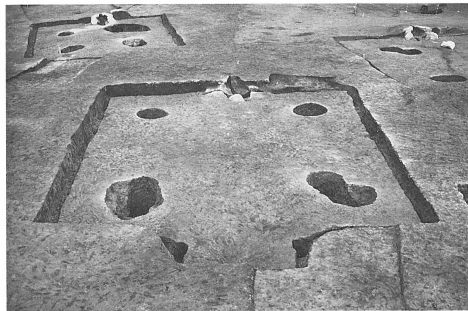
竖穴住居35
