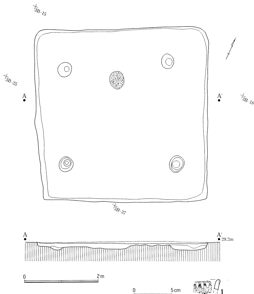
第43図 020住居跡実測図
