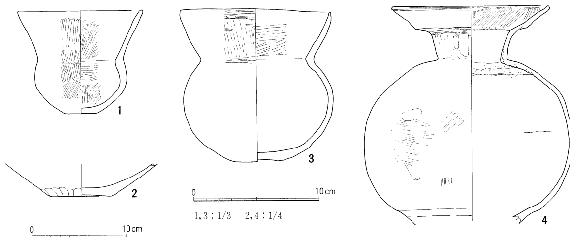
第16図 050住居跡実測図
