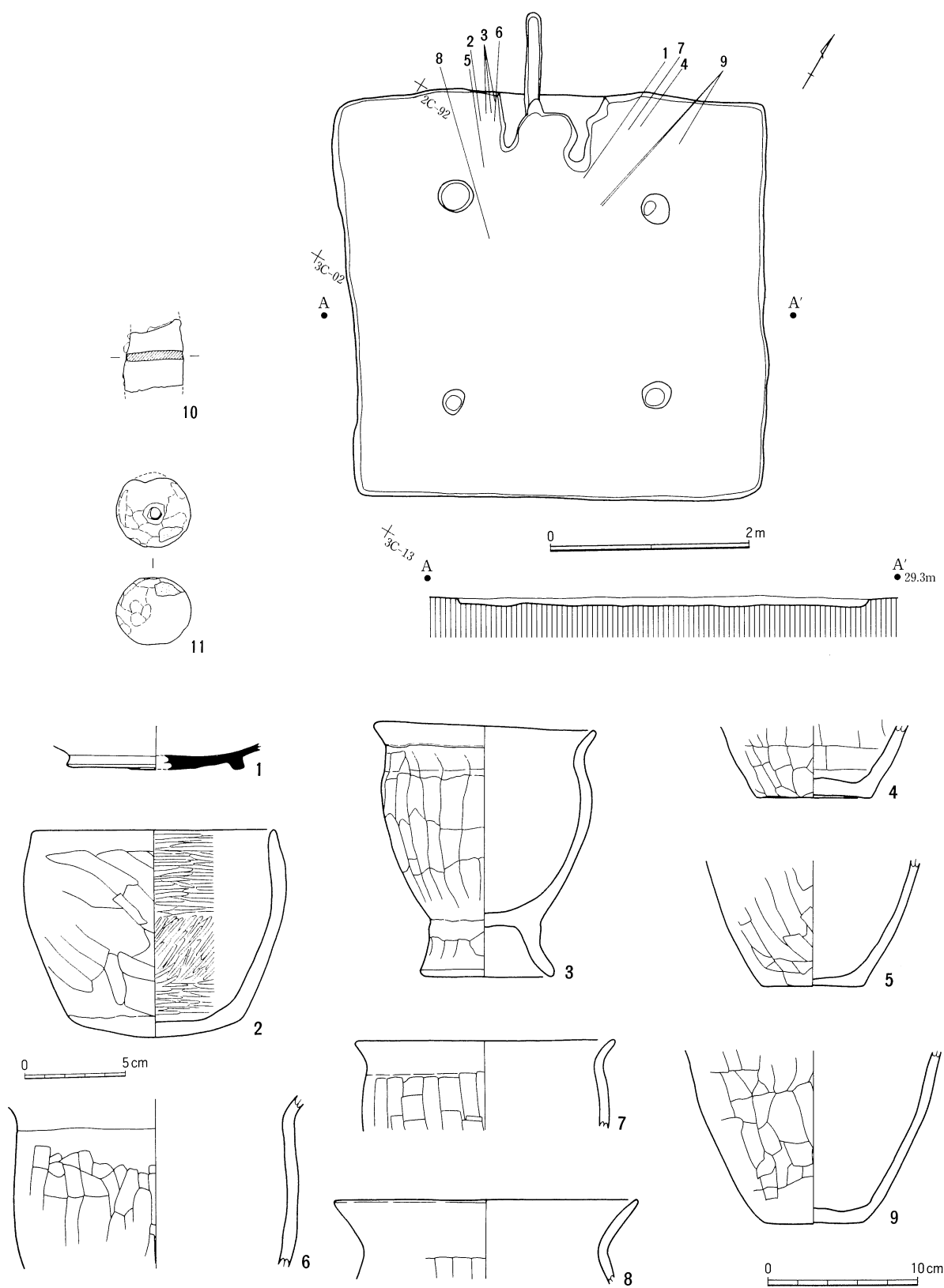
第69図 014住居跡実測図
