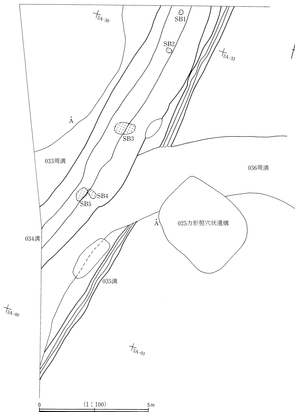
第80図 034溝・035溝実測図
