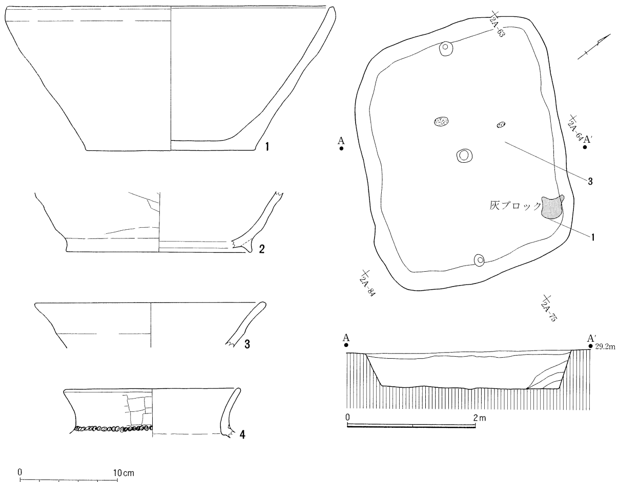
第78図 025方形竪穴状遺構実測図
