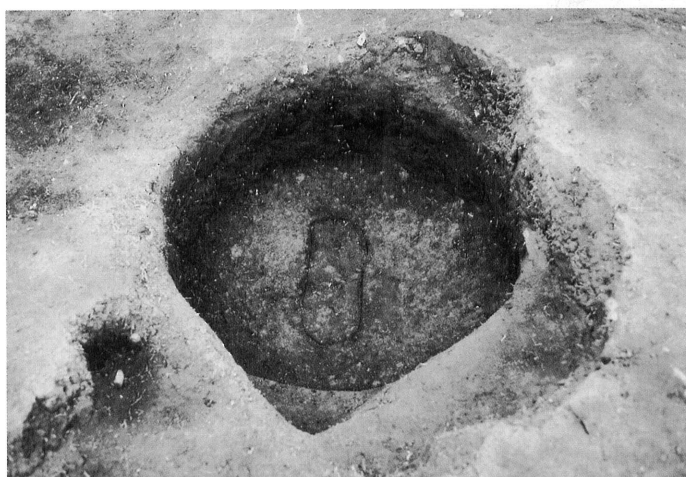
SB-02柱痕検出状況
