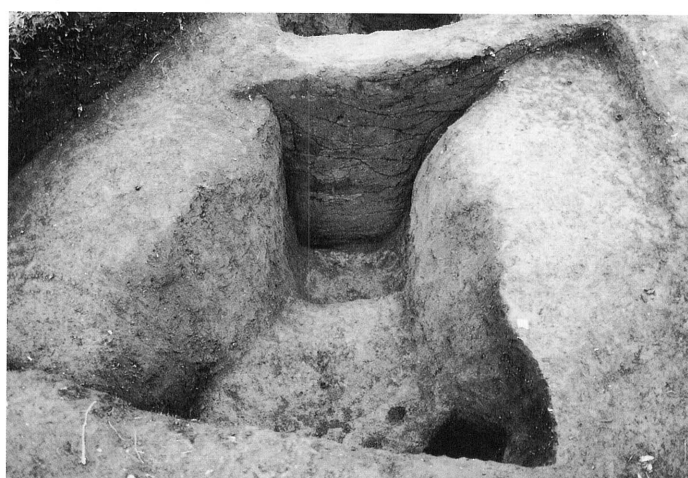
SX-15セクション F-F'
