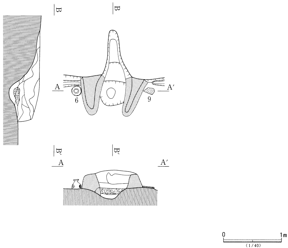
第186図 7号住居跡(1)
