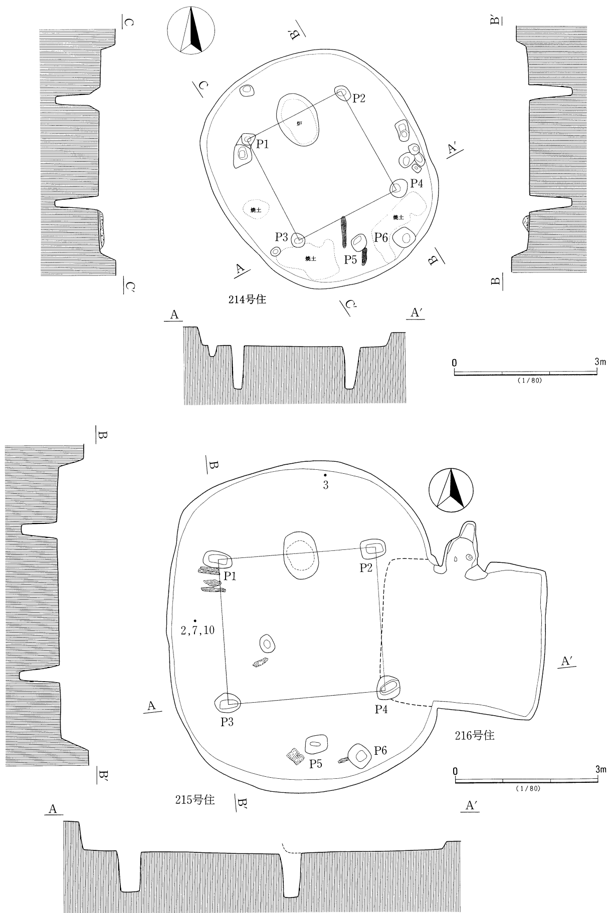
第147図 214号住居跡・215号住居跡(1)
