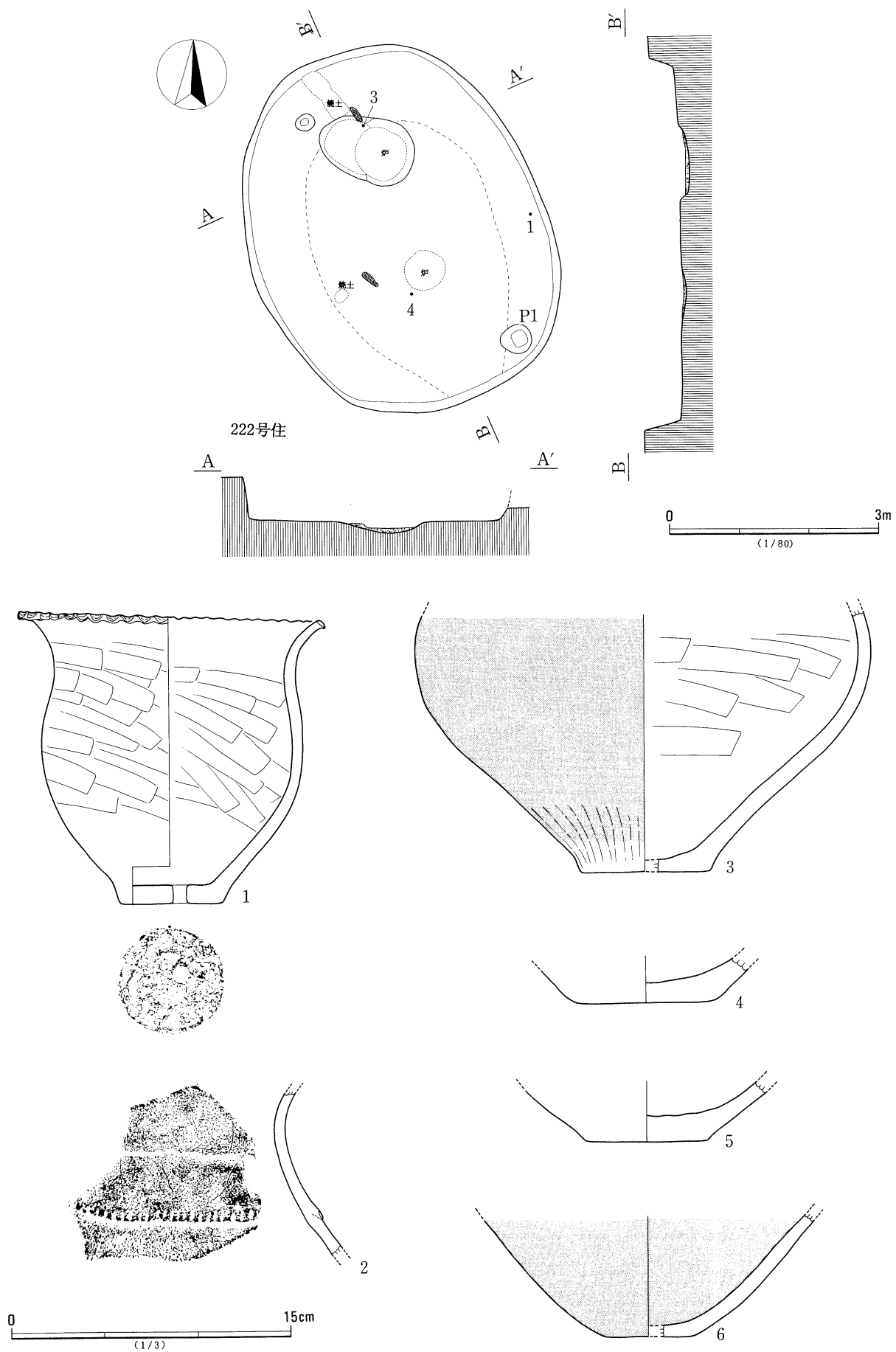
第155図 222号住居跡
