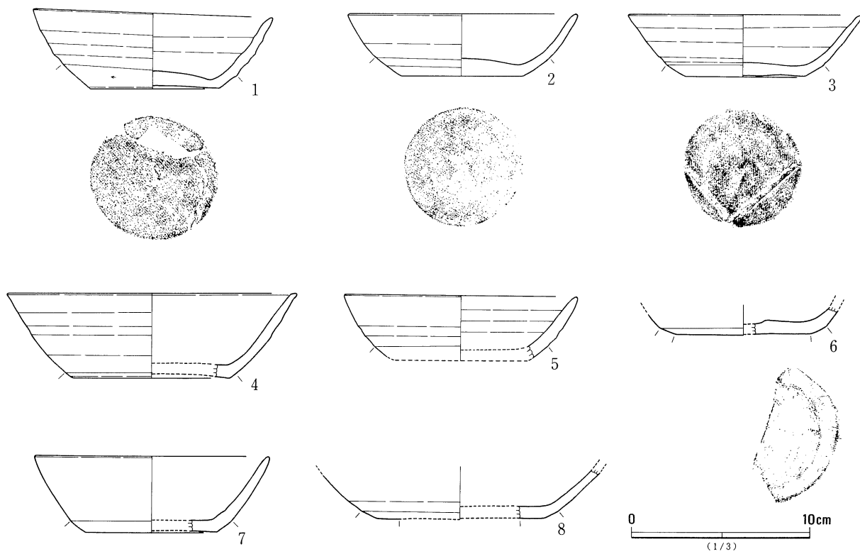
第174図 5号住居跡(1)
