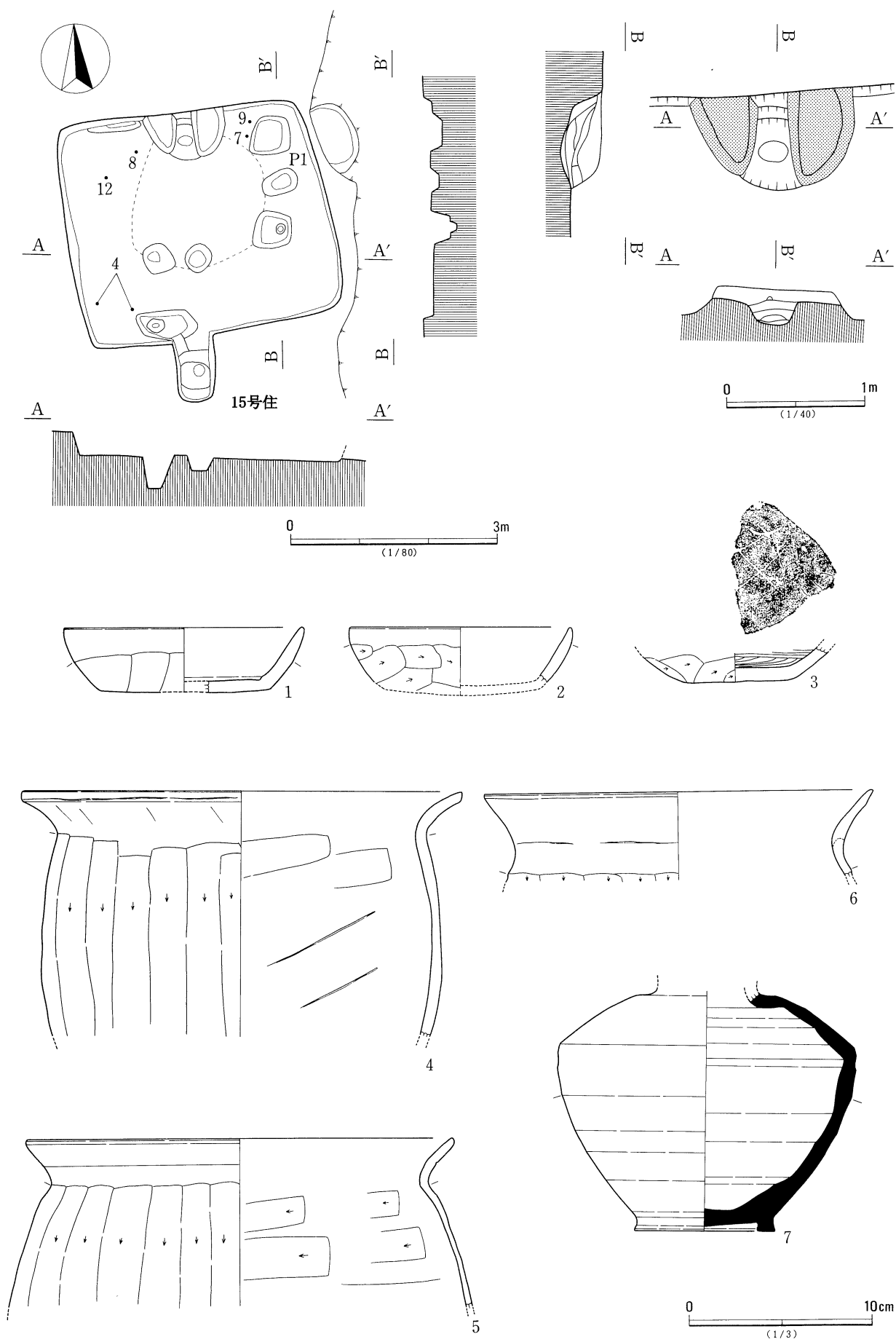
第203図 15号住居跡(1)
