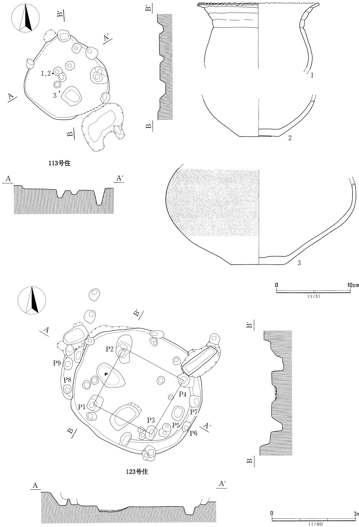
第130図 113号・123号住居跡
