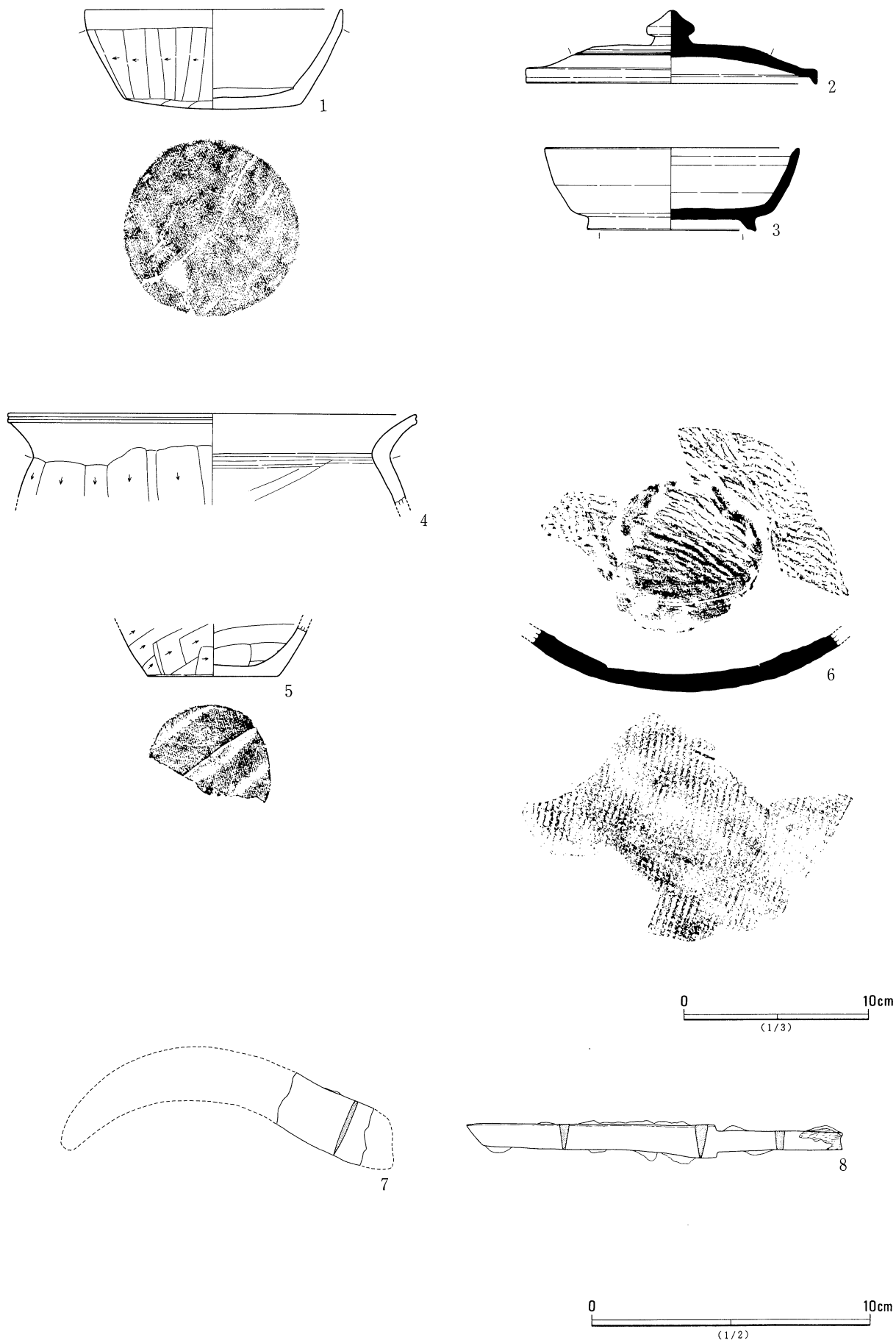
第201図 12号住居跡(2)
