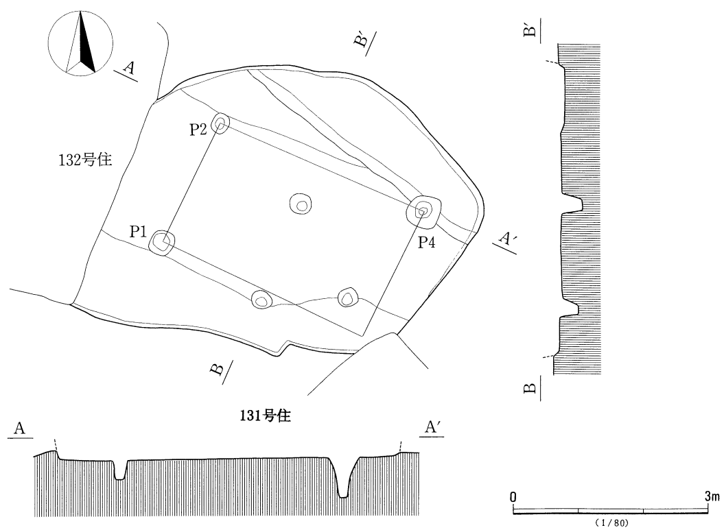
第131図 129号・131号住居跡
