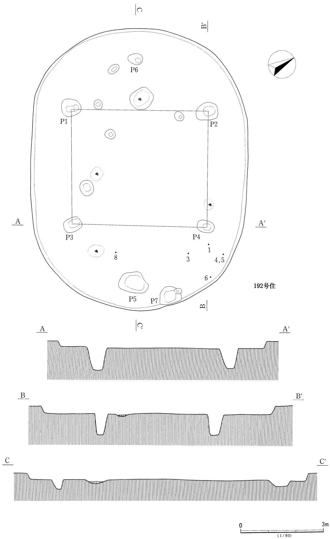
第140図 192号住居跡(1)
