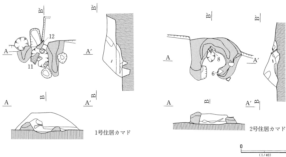
第166図 1号・2号・3号住居跡(1)
