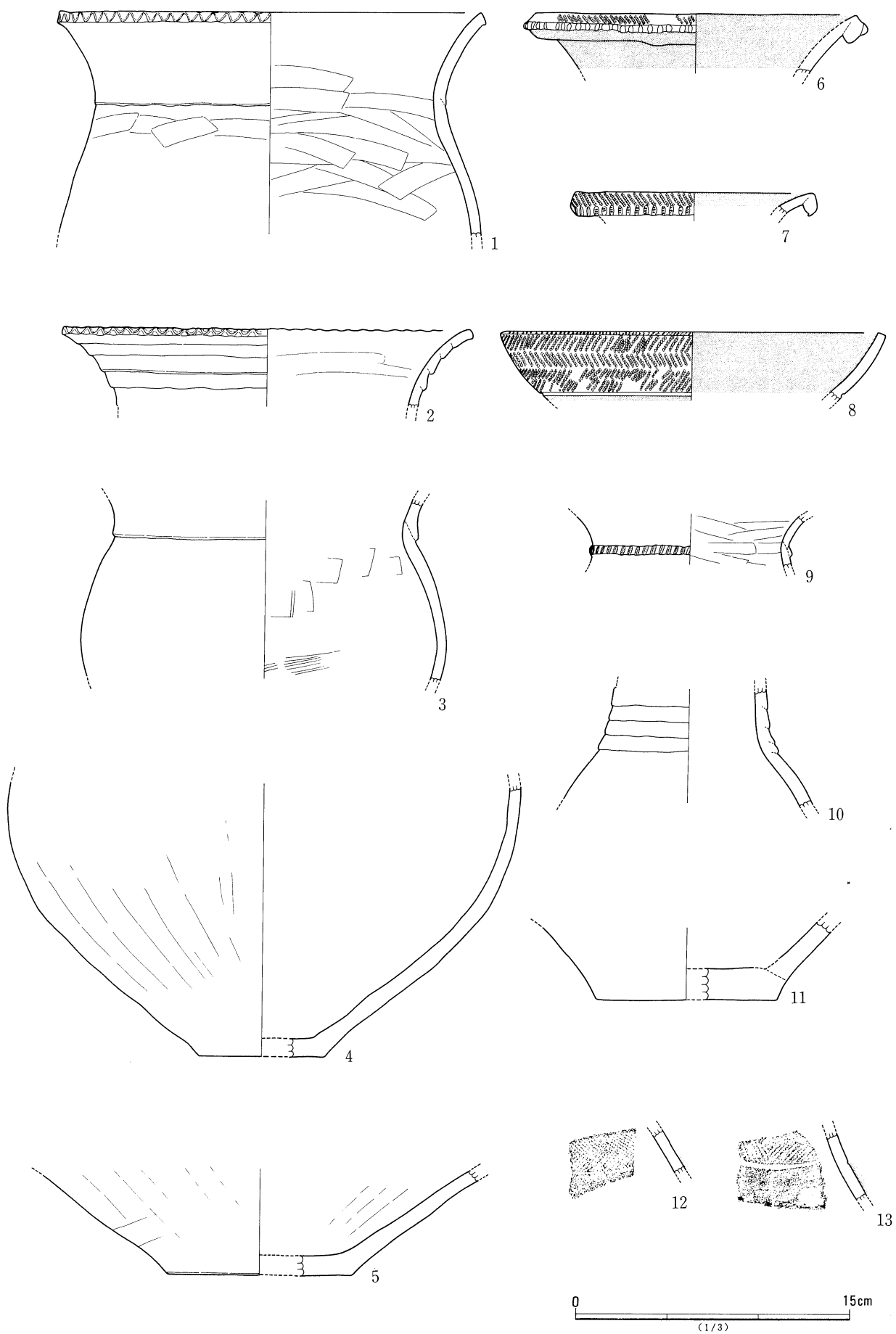
第148图 215号住居跡(2)
