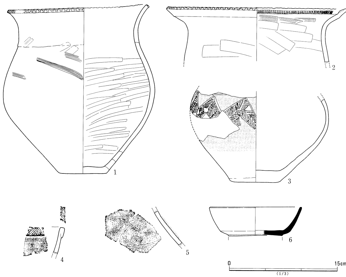
第157図 224号住居跡
