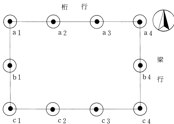
掘立柱建物跡凡例
