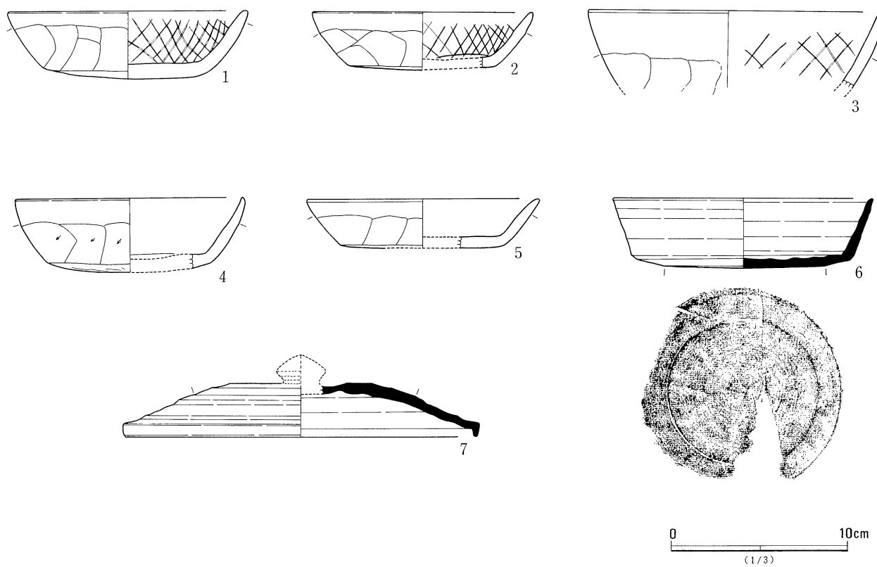
第192図 9号住居跡(1)
