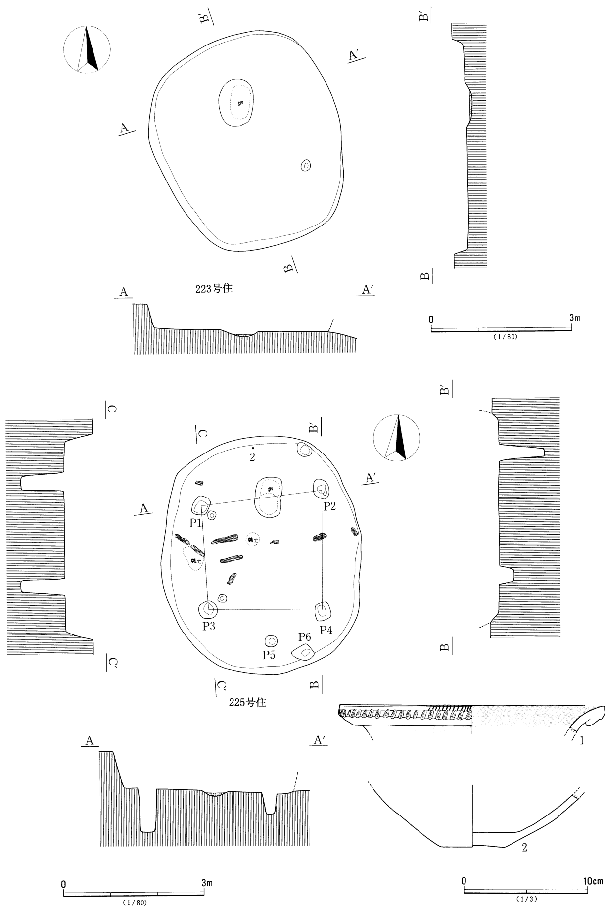
第156図 223号・225号住居跡
