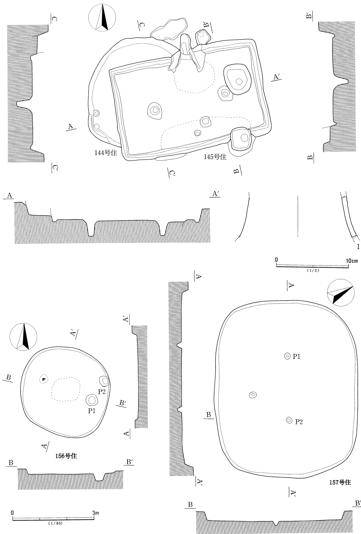
第132図 144号・156号・157号住居跡
