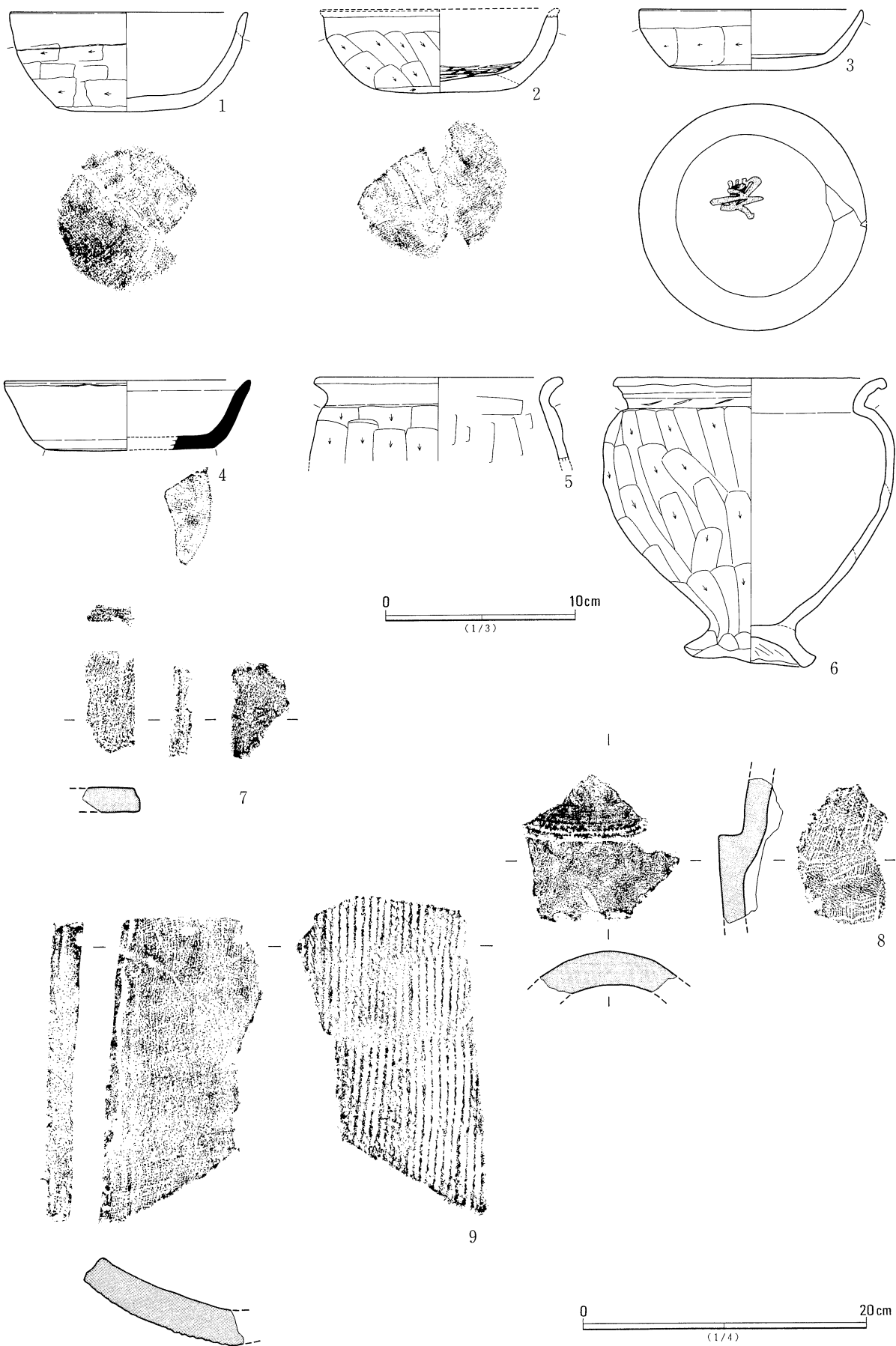
第187図 7号住居跡(2)
