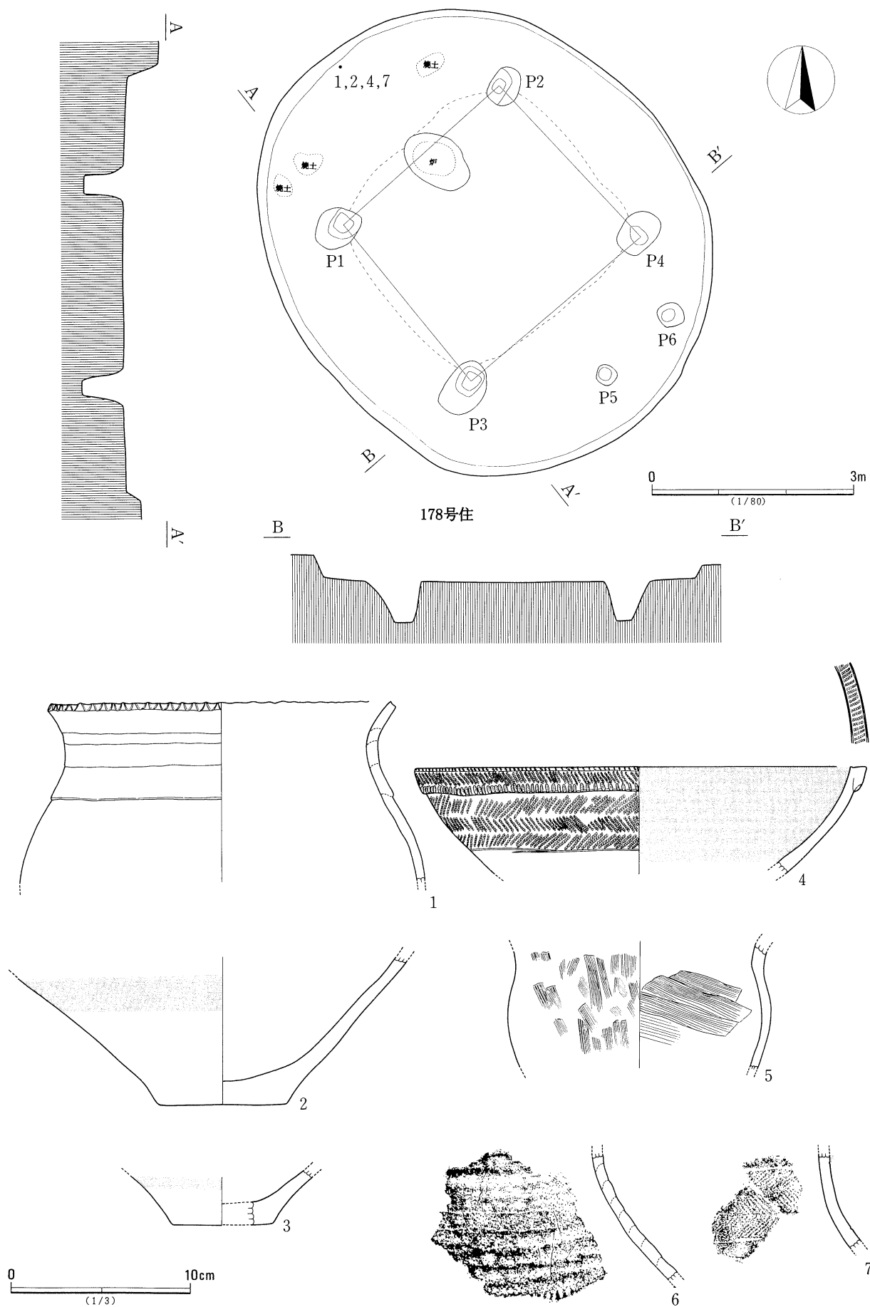
第136図 178号住居跡
