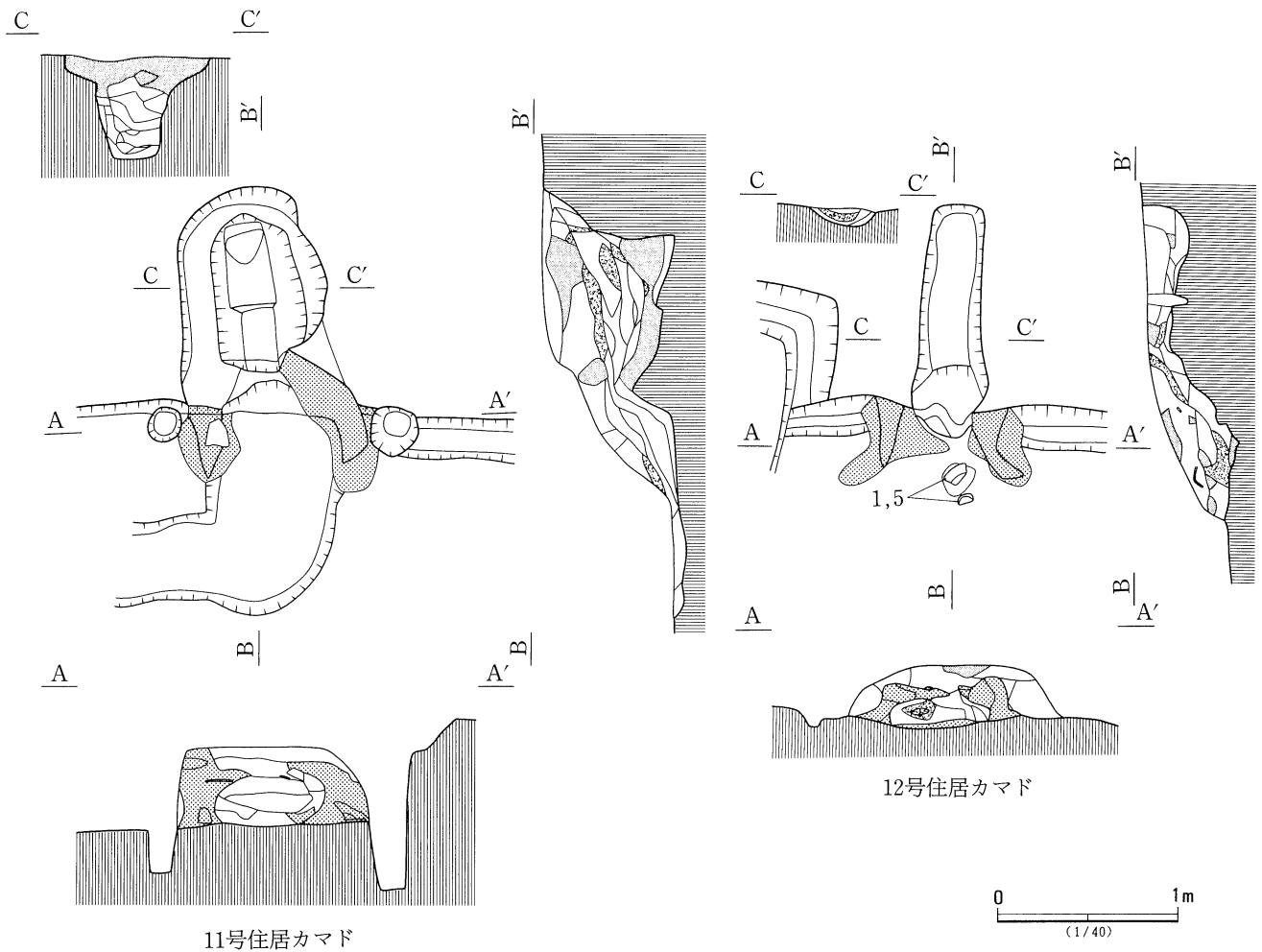
第198図 11号・12号住居跡(1)
