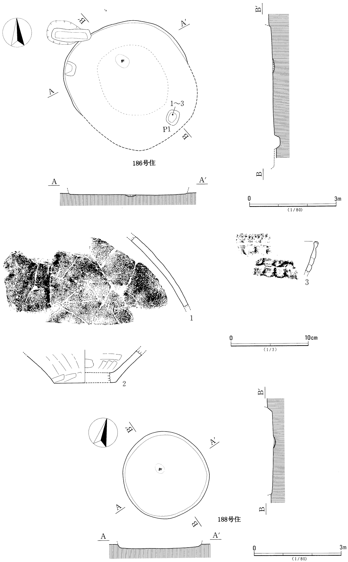
第137図 186号・188号住居跡
