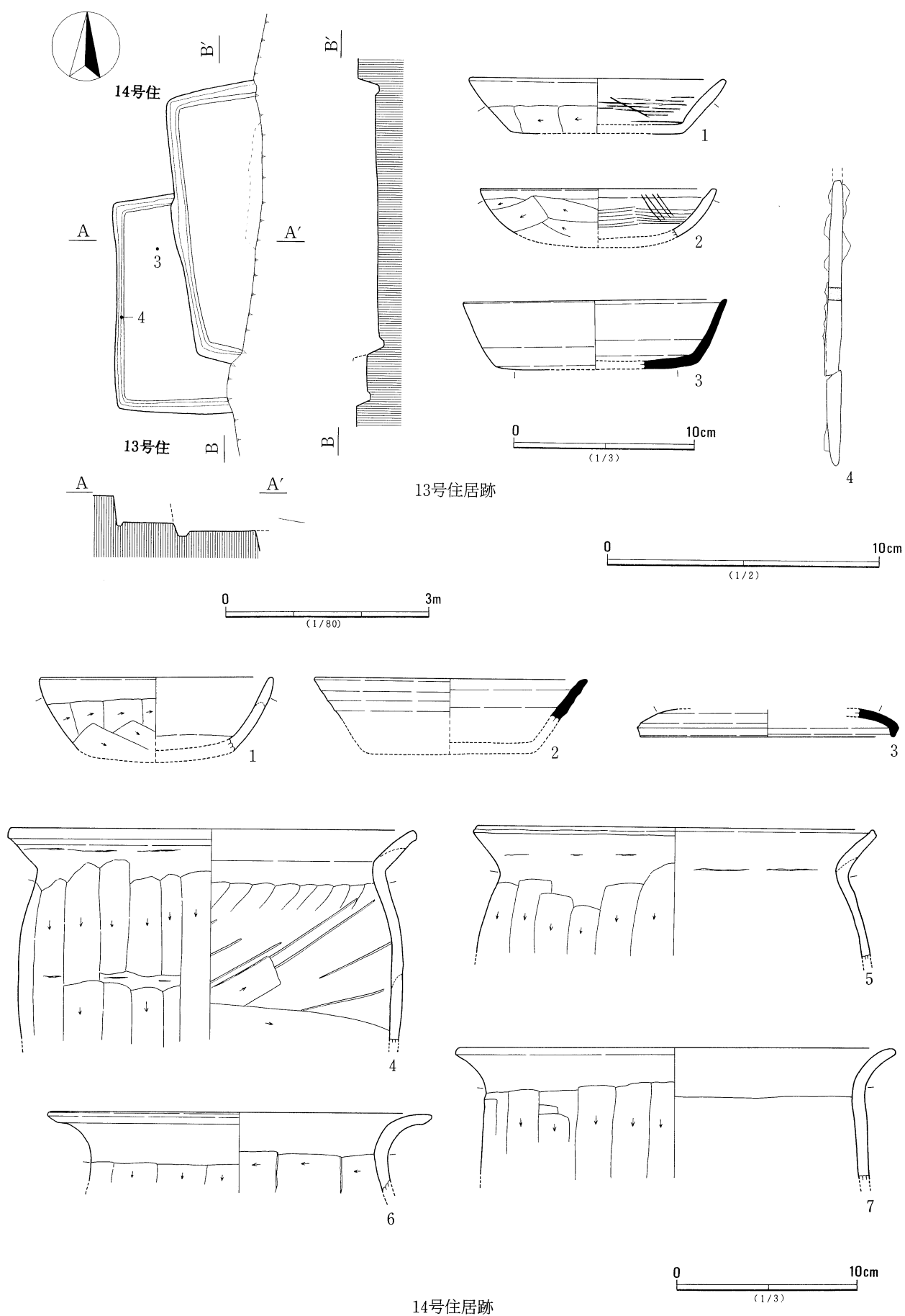
第202図 13号・14号住居跡
