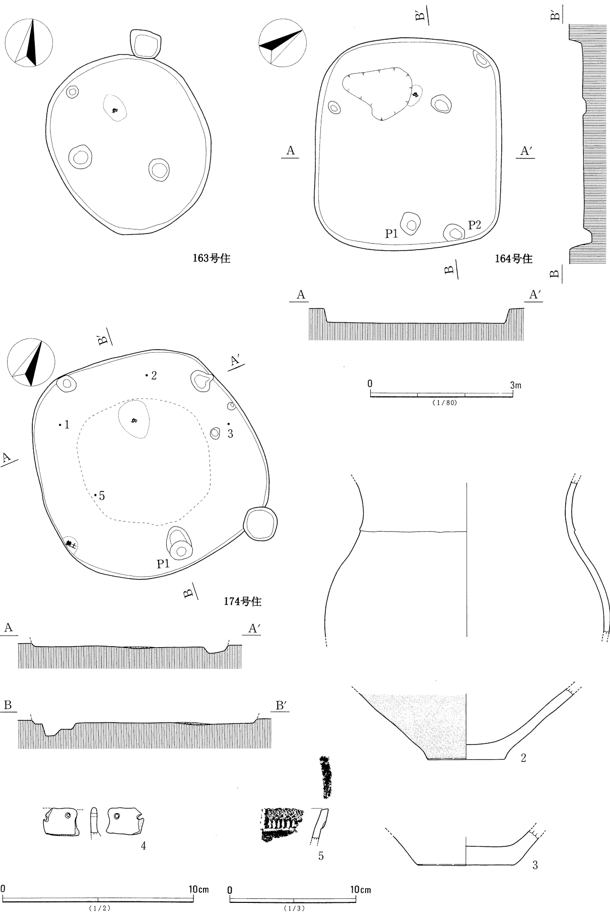
第134図 163号・164号・174号住居跡
