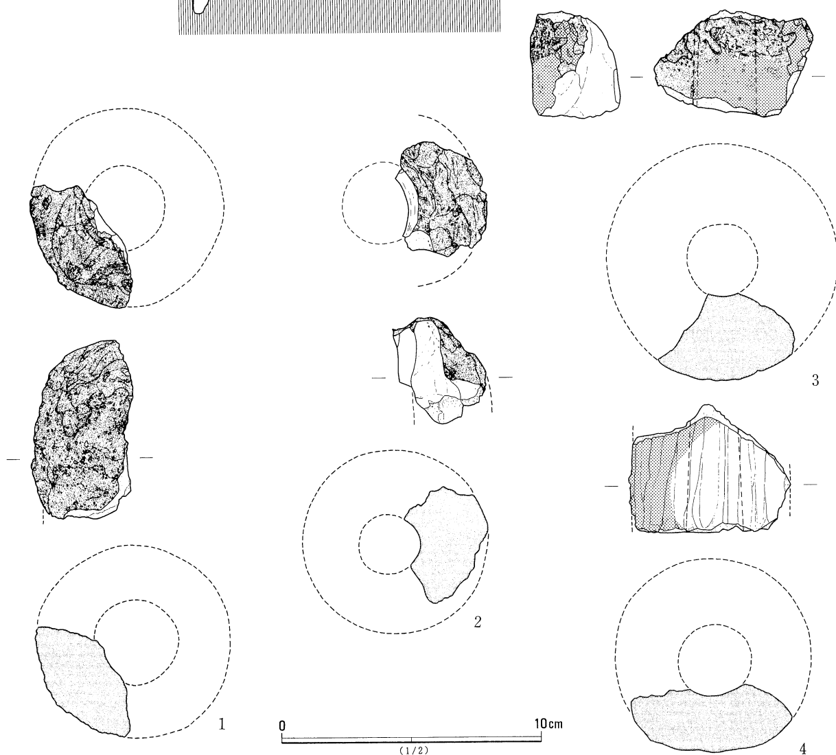
第501図 499号鍛冶遺構
