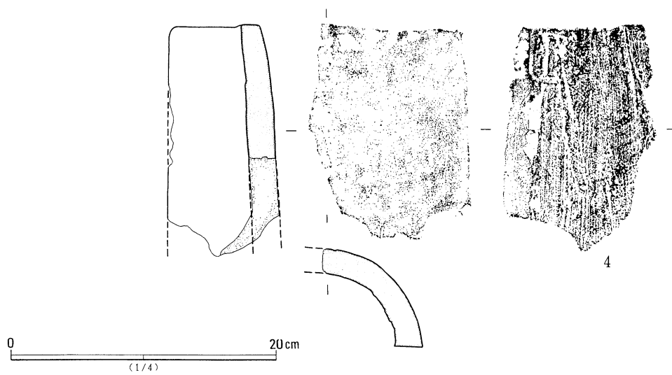
第505図 506号掘立柱建物跡(1)
