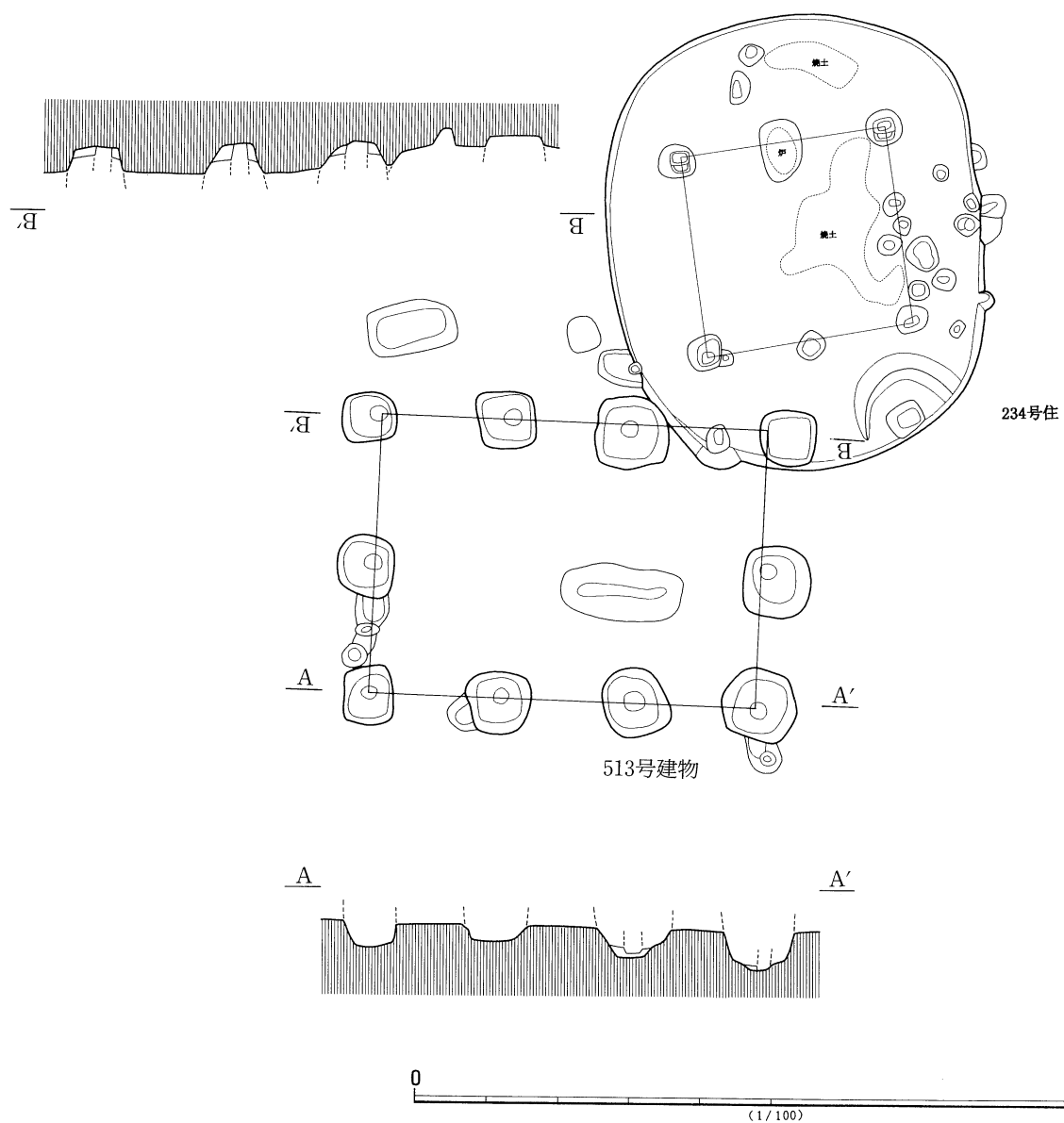
第511図 513号掘立柱建物跡
