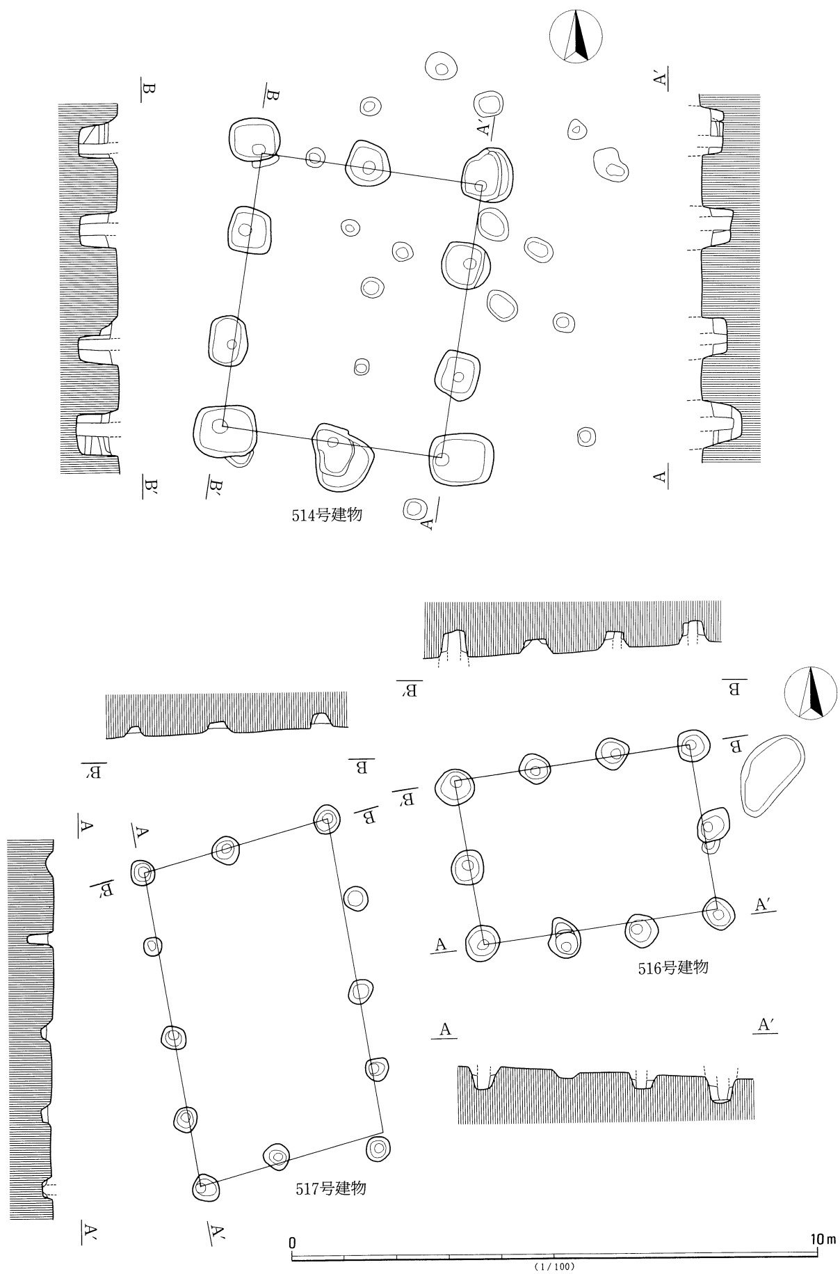
第512図 514号・516号・517号掘立柱建物跡
