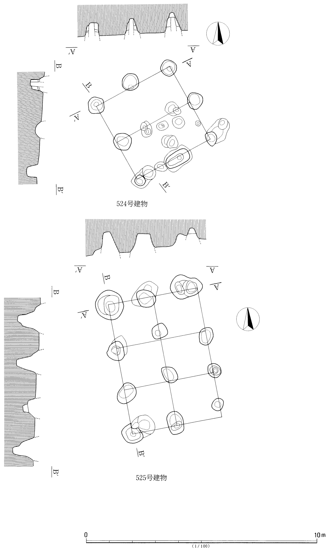
第517図 524号・525号掘立柱建物跡
