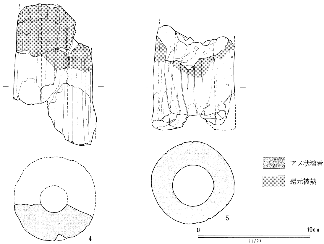
第483図 373号鍛冶遺構(1)
