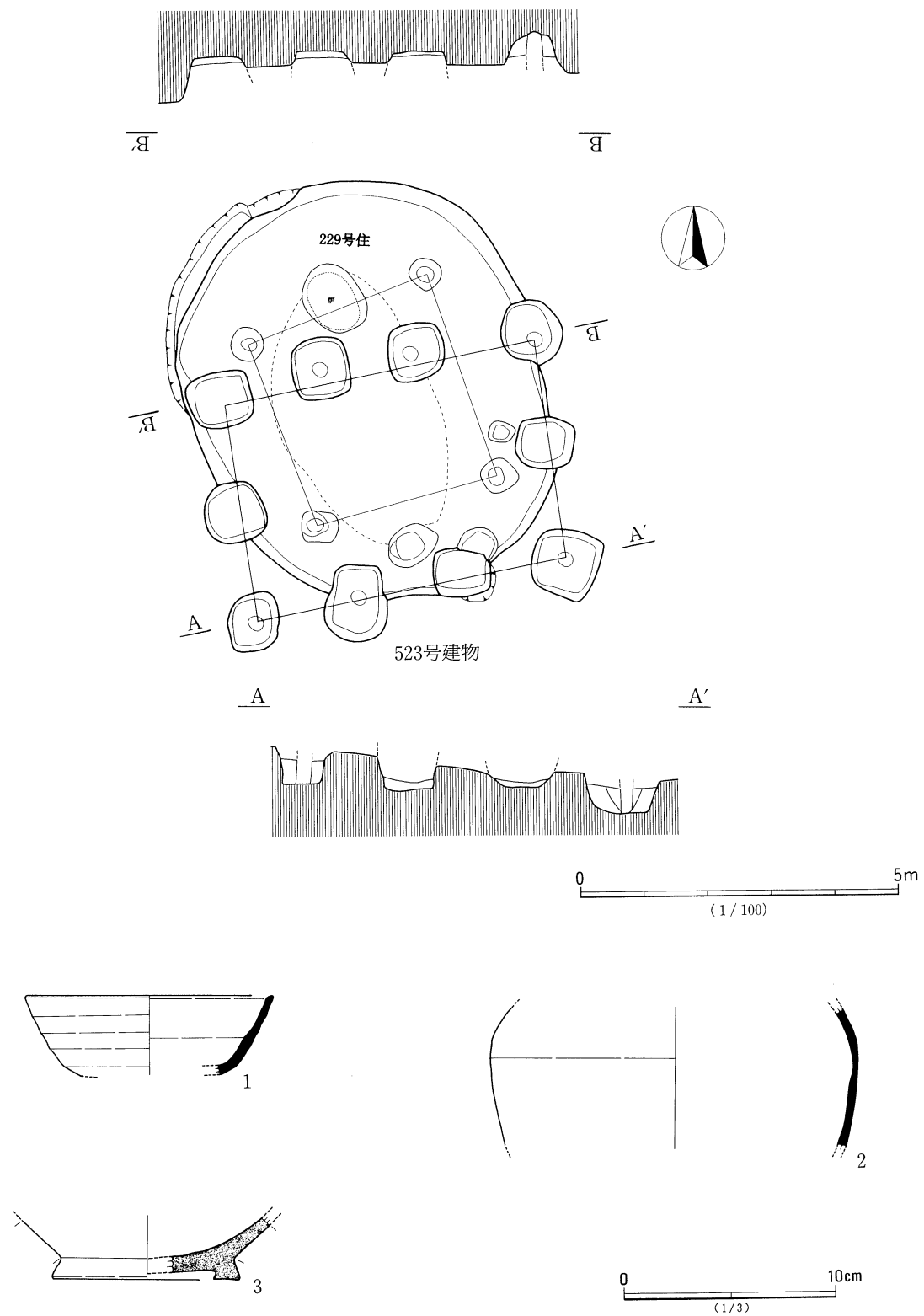
第516図 523号掘立柱建物跡
