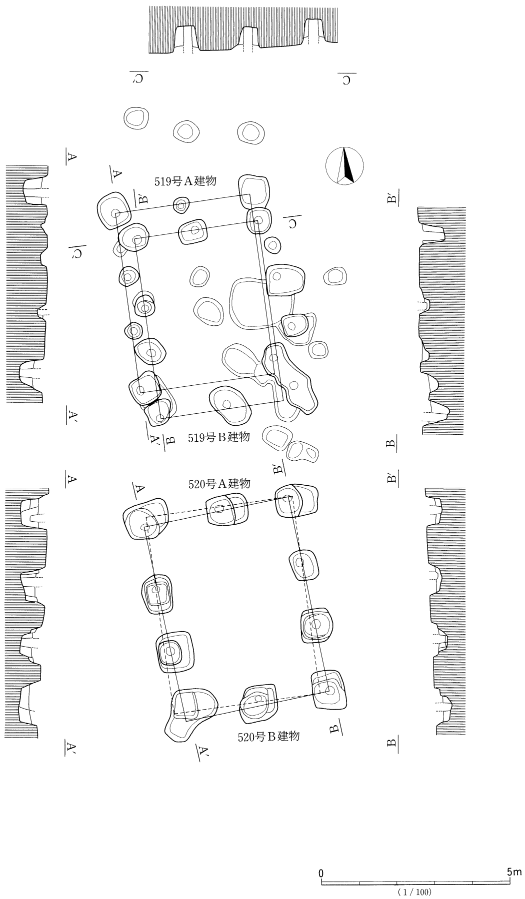
第514図 519号・520号掘立柱建物跡
