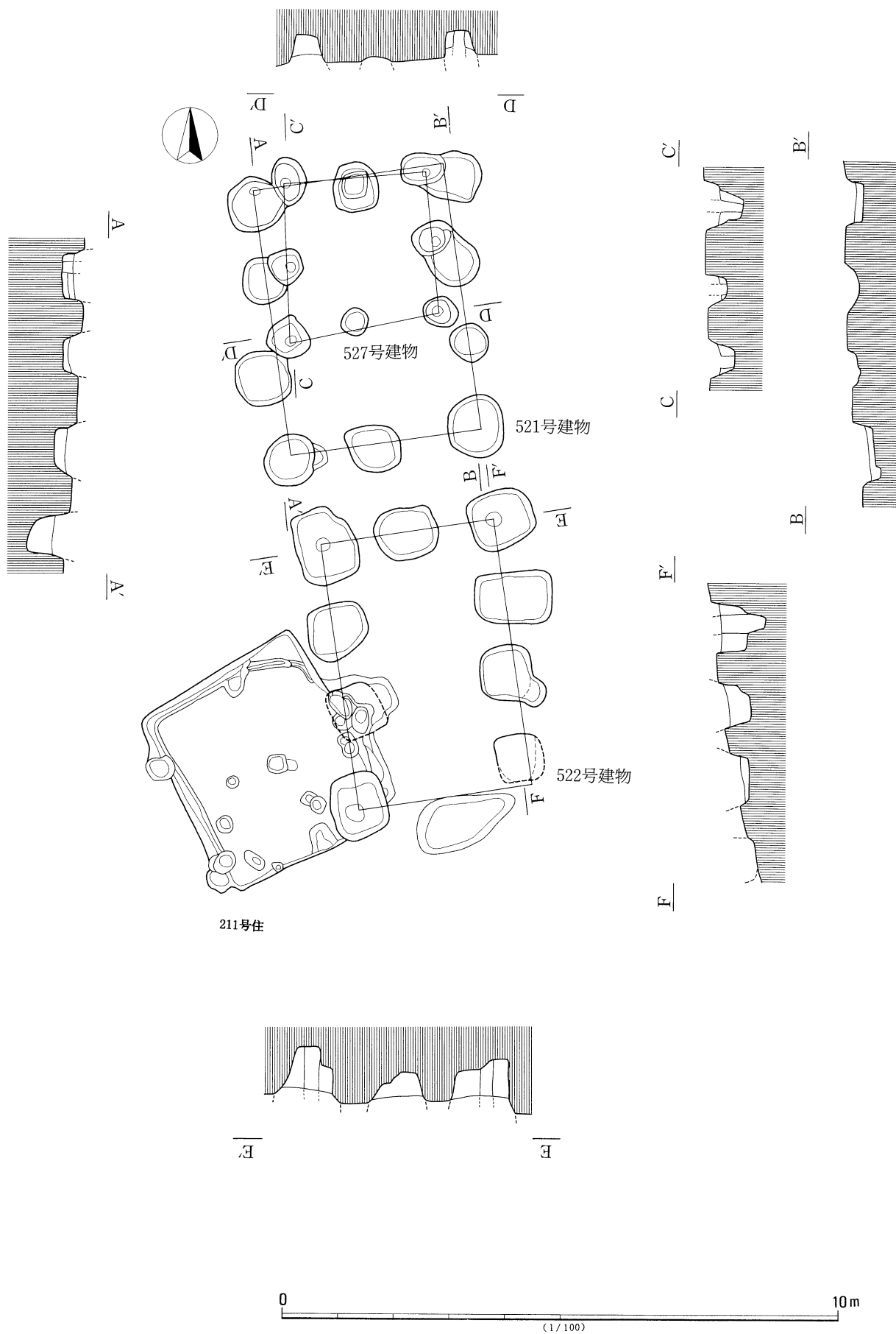
第515図 521号・522号・527号掘立柱建物跡
