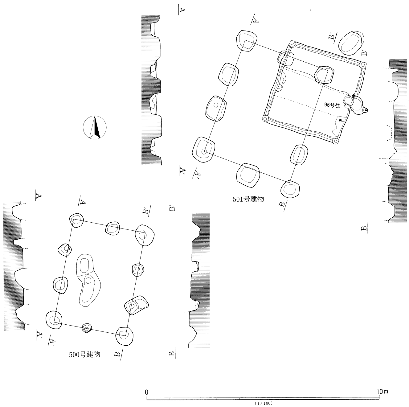
第502図 500号・501号掘立柱建物跡
