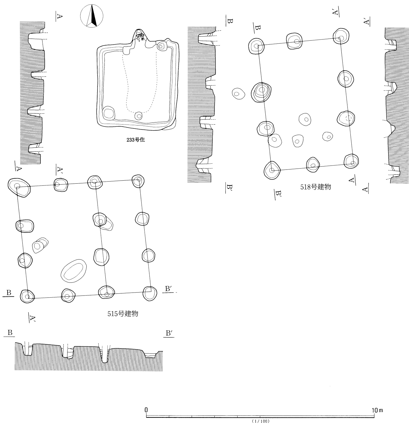
第513図 515号・518号掘立柱建物跡
