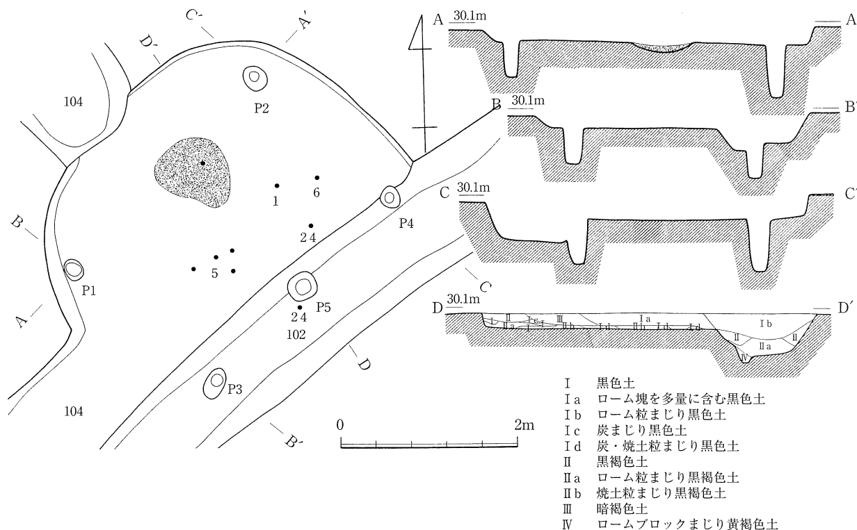
第4図 201号住居跡
