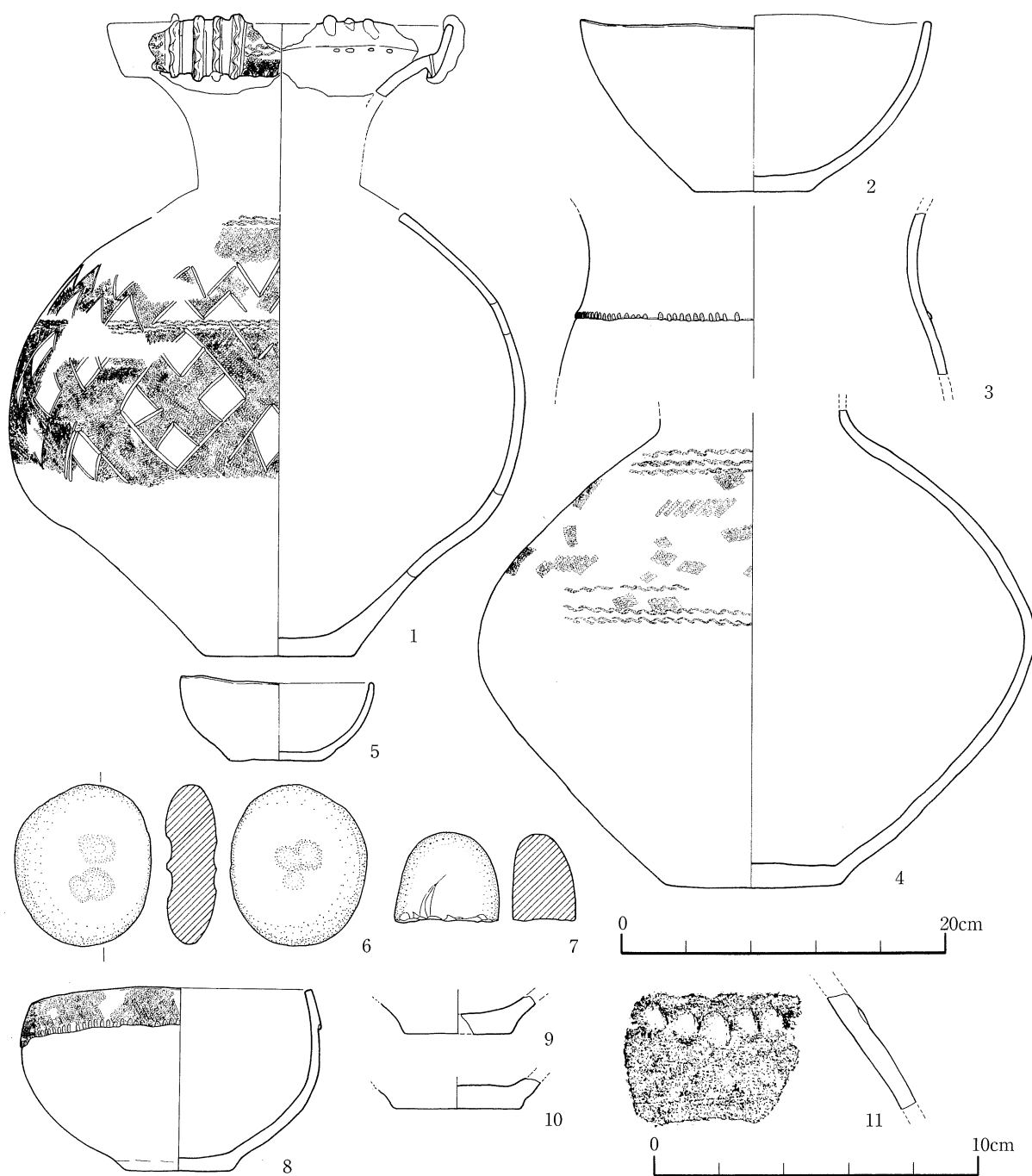
第9図 203(1~7)・204(8~10)出土遺物
