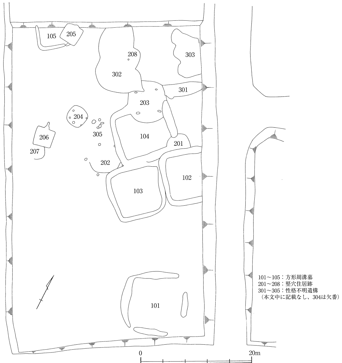
第3図 南祇園原遺跡全体図 (1/400)
