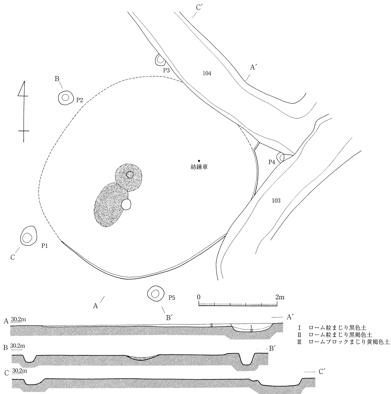
第5図 202号住居跡
