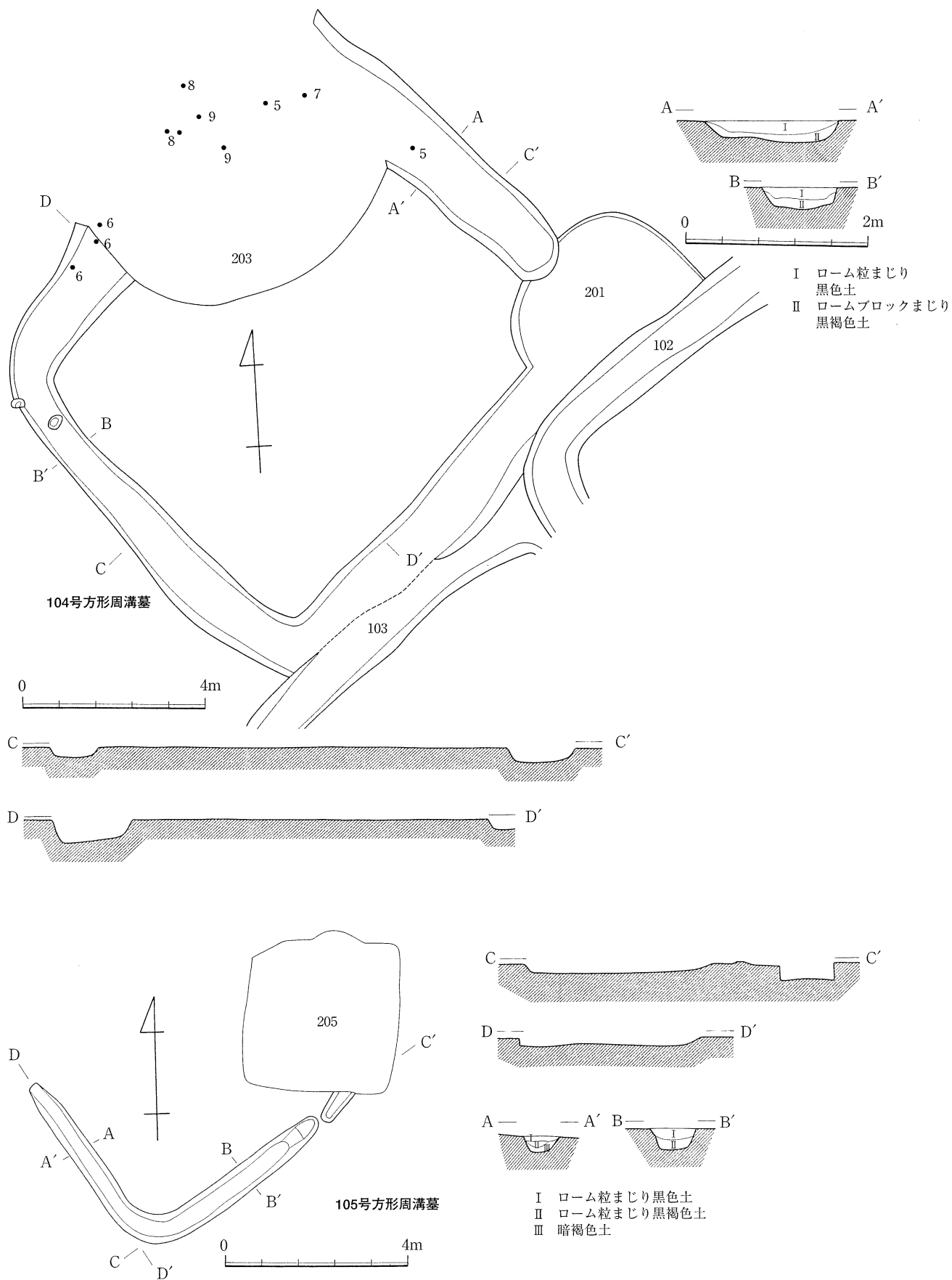
第18図 104号(上)、105号方形周溝墓 (水準線はいずれも30.1m)
