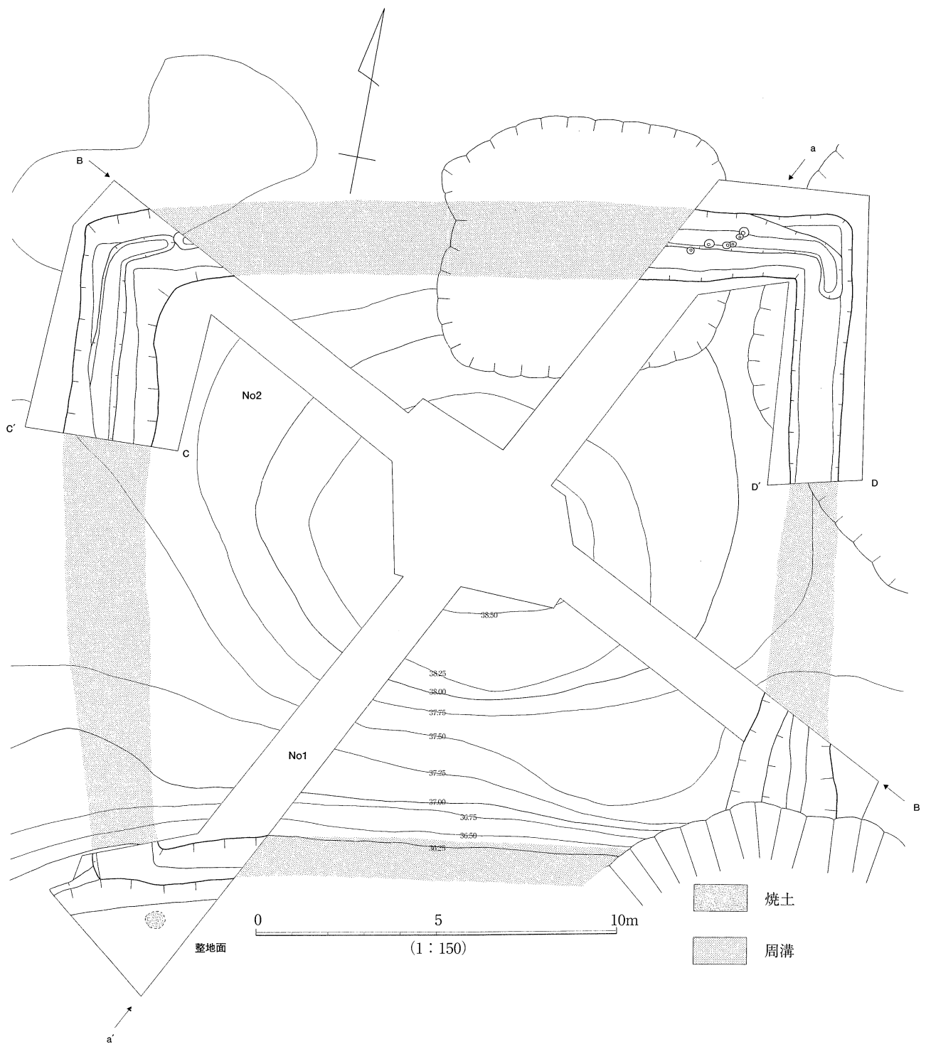
第25図 持塚5号墳トレンチ配置図 (Noはトレンチ番号)
