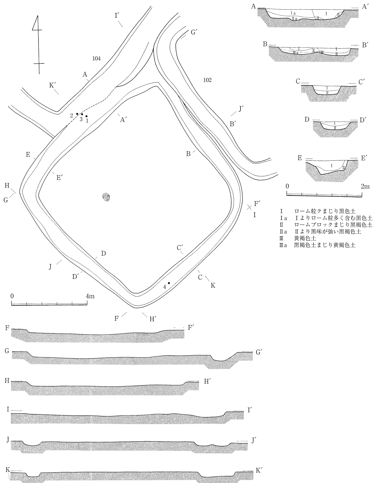
第17図 103号方形周溝墓 (水準線はいずれも30.1m)
