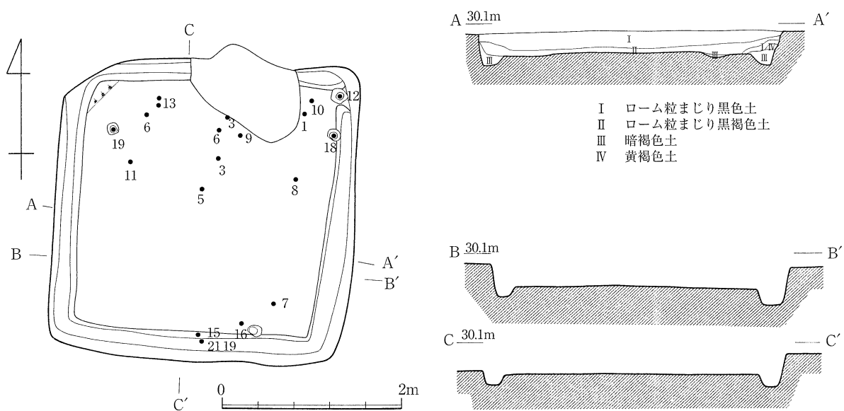
第10図 205号住居跡
