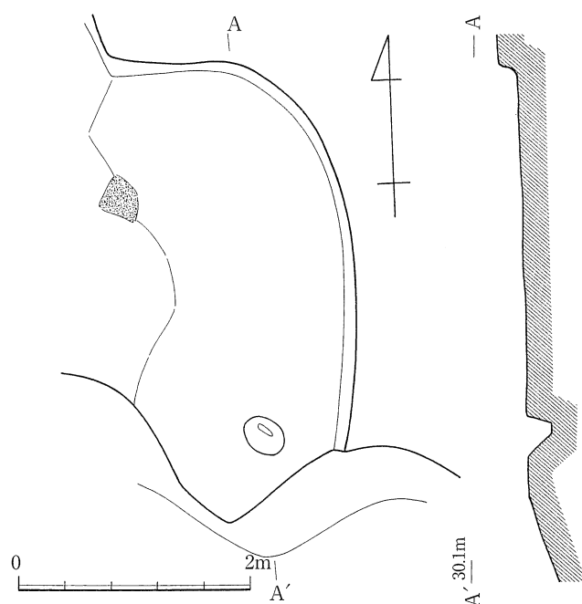
第14図 208号住居跡
