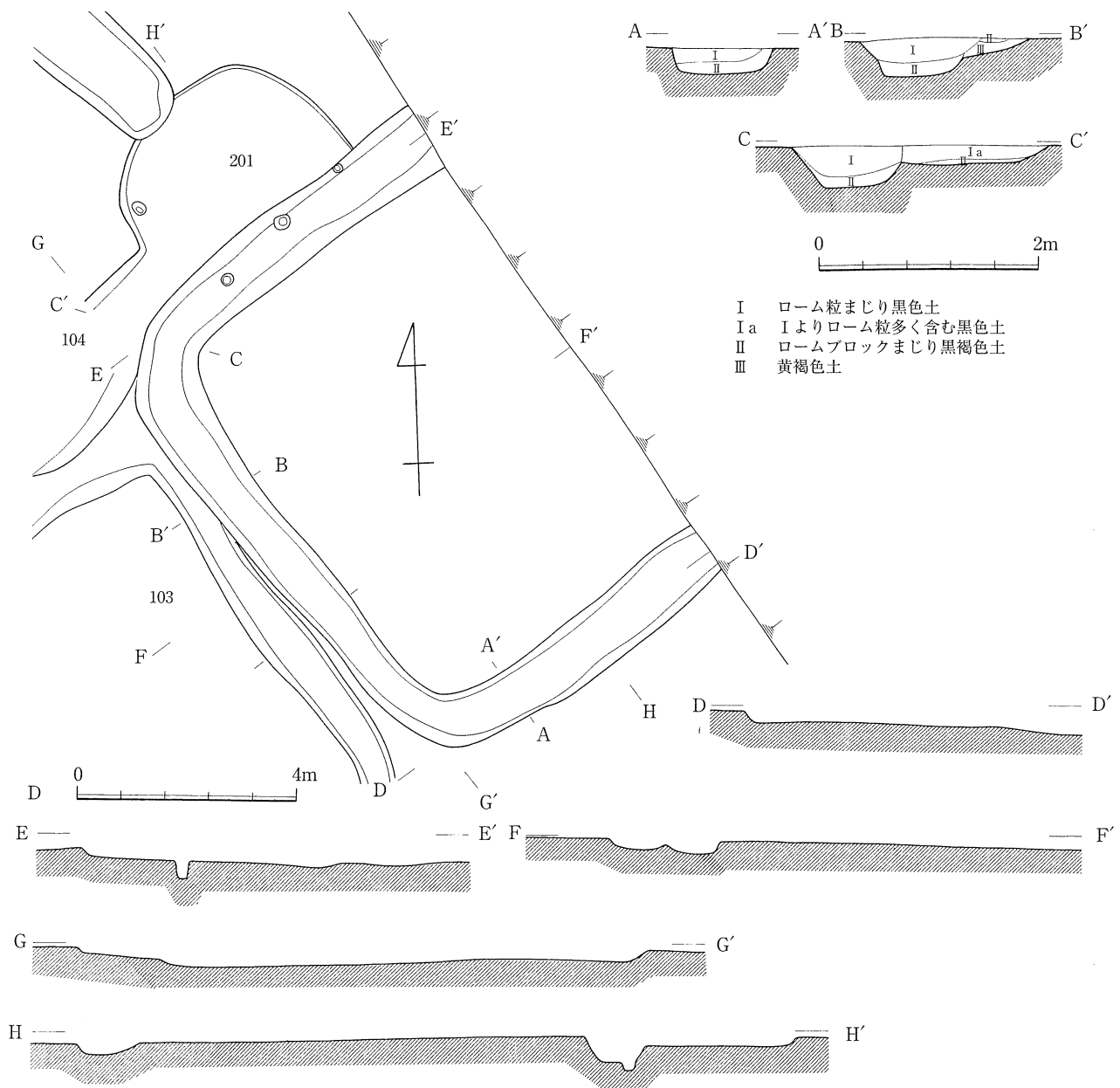
第16図 102号方形周溝墓 (水準線はいずれも30.1m)
