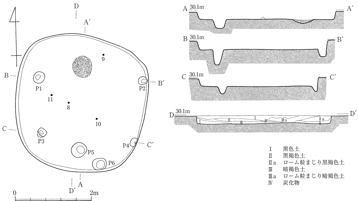
第8図 204号住居跡
