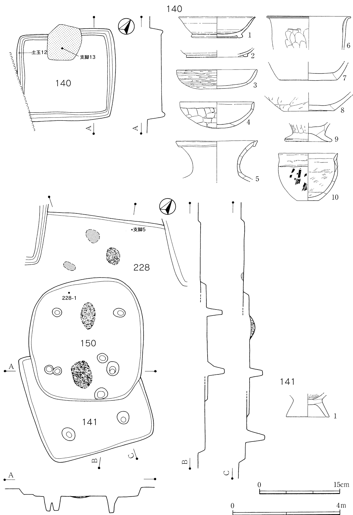
第73図 140・141・150・228号住居跡と140・141号住居跡出土土器
