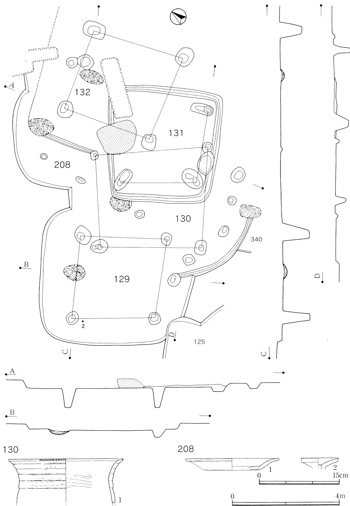
第67図 129～132・208号住居跡と130・208号住居跡出土土器
