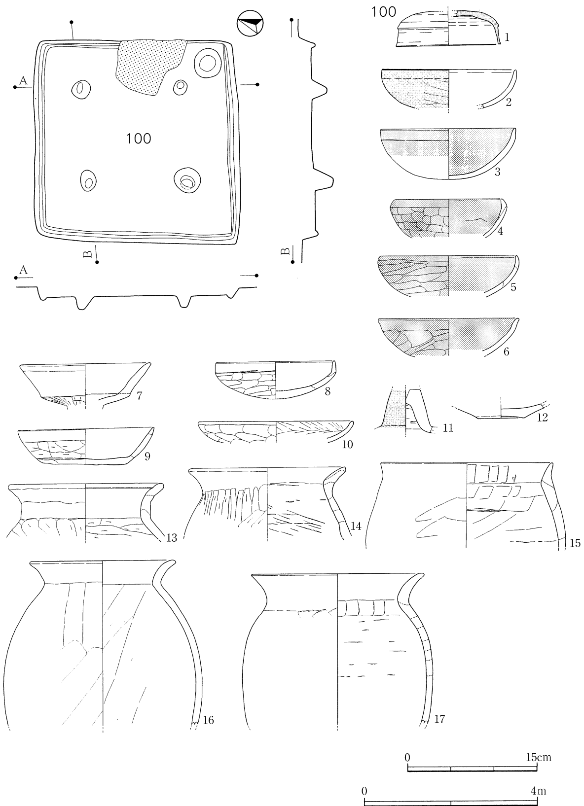
第53図 100号住居跡と出土土器
