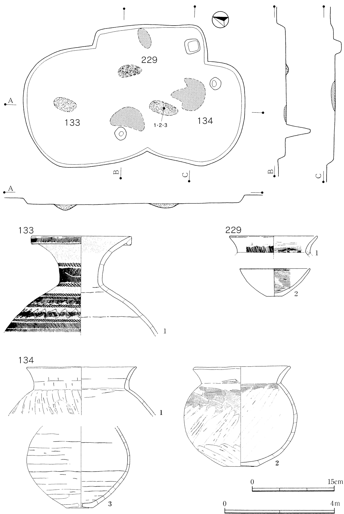
第69図 133・134・229号住居跡と出土土器
