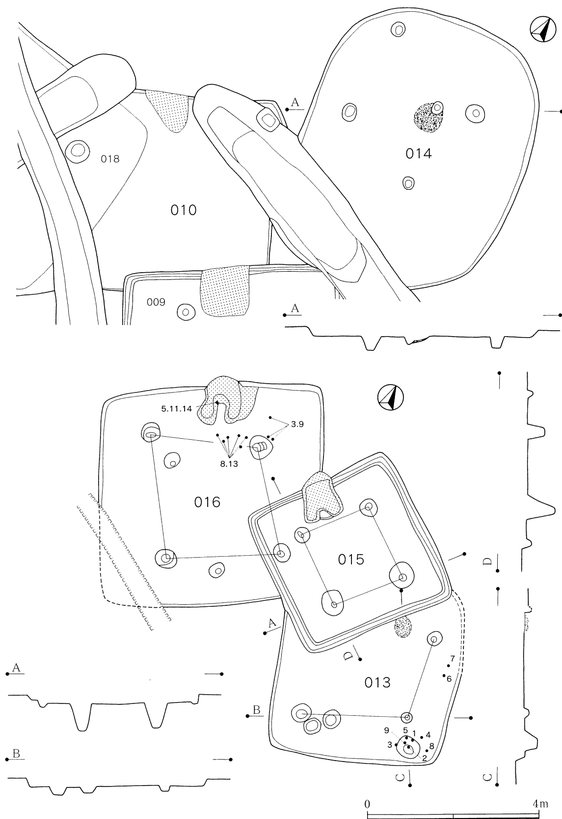
第16図 010・013~016号住居跡
