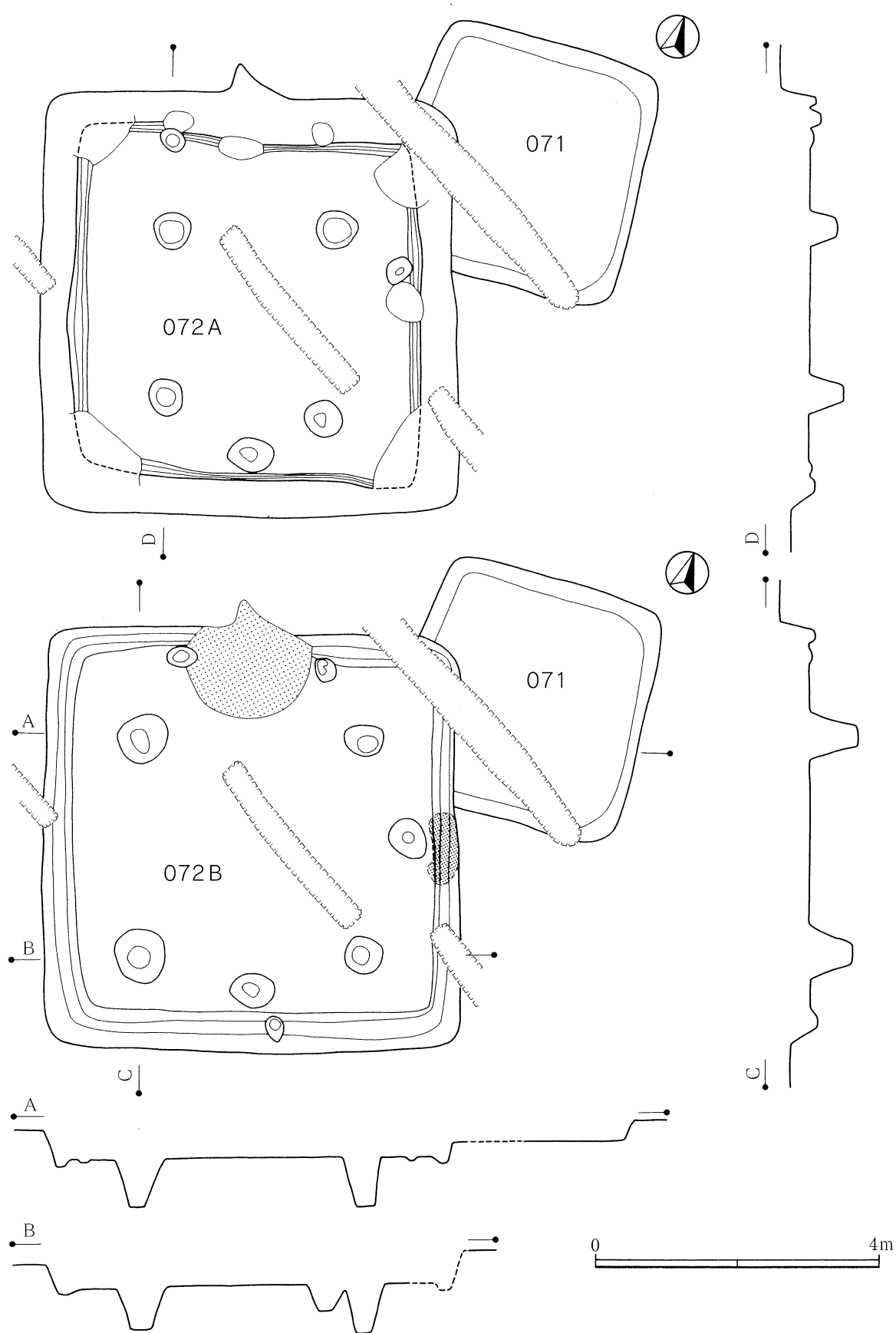
第44图 071·072A·B号住居跡
