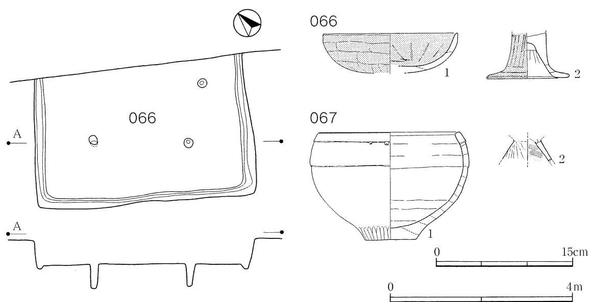
第42図 066号住居跡と061・065～067号住居跡出土土器
