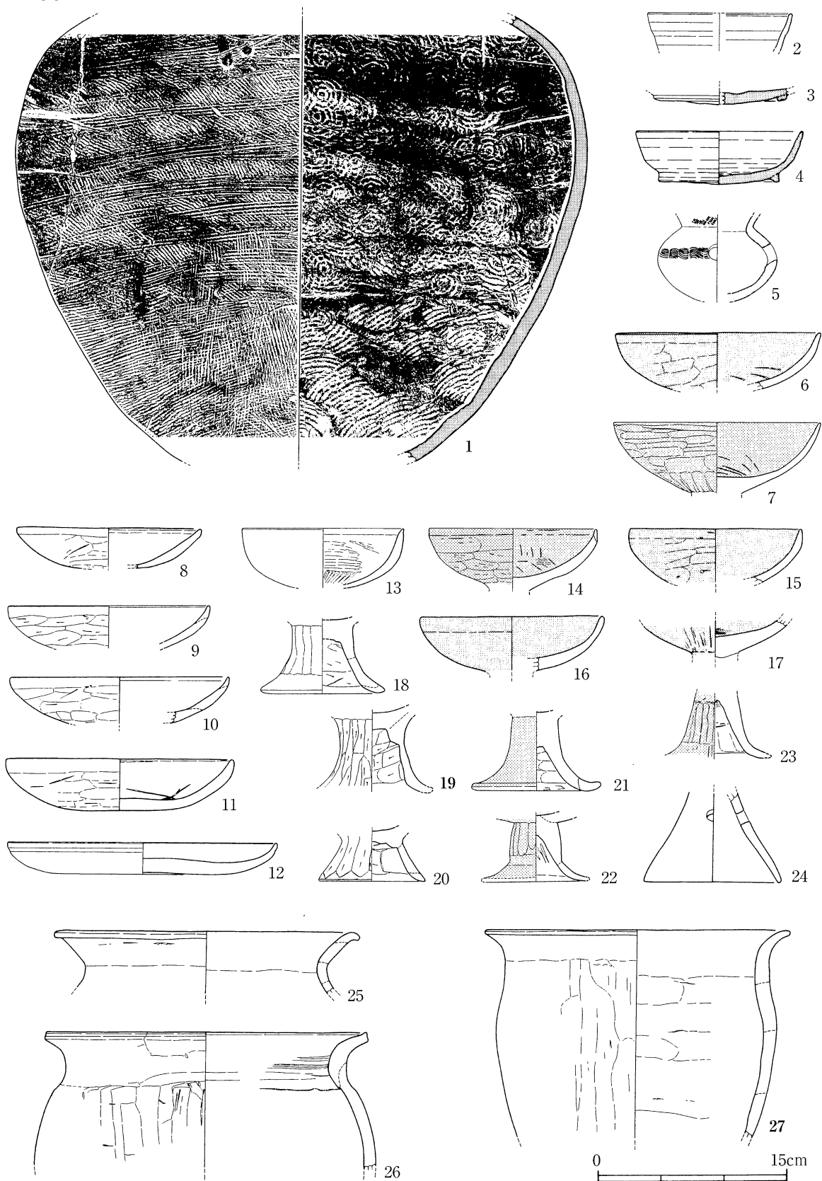
第27图 034号住居跡出土土器
