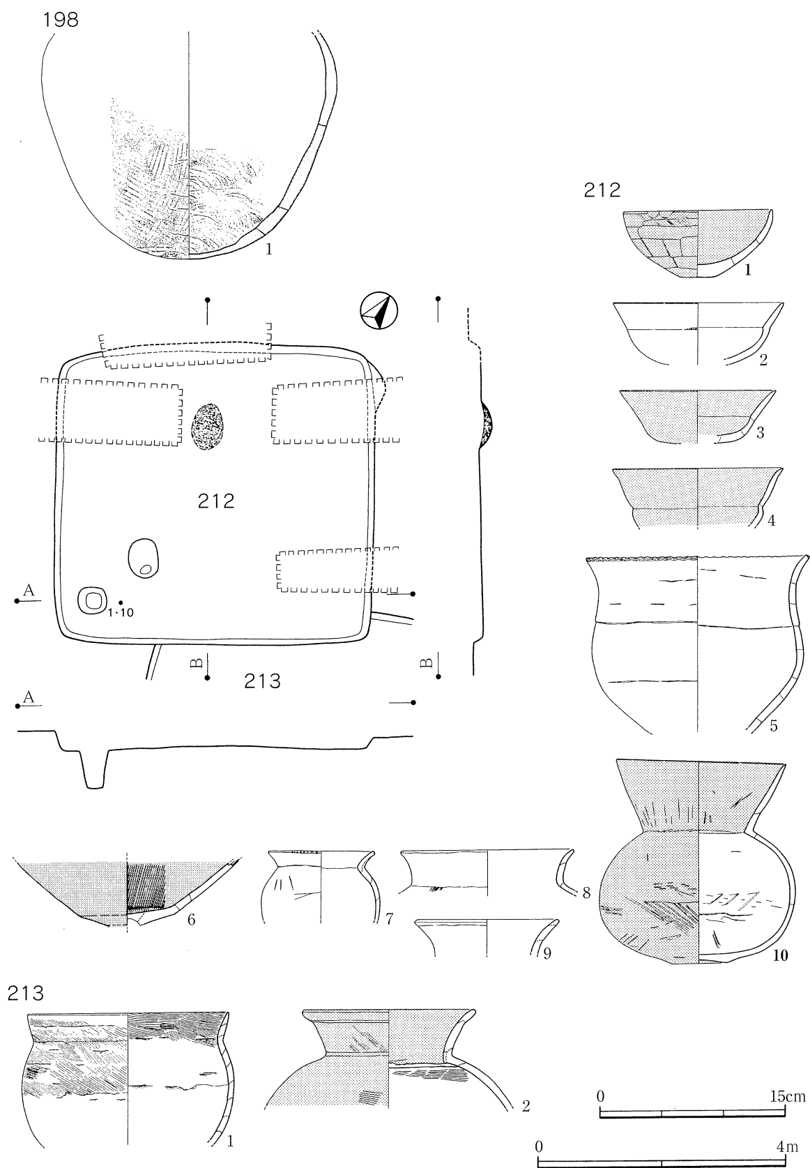
第97図 212・213号住居跡と198・212・213号住居跡出土土器
