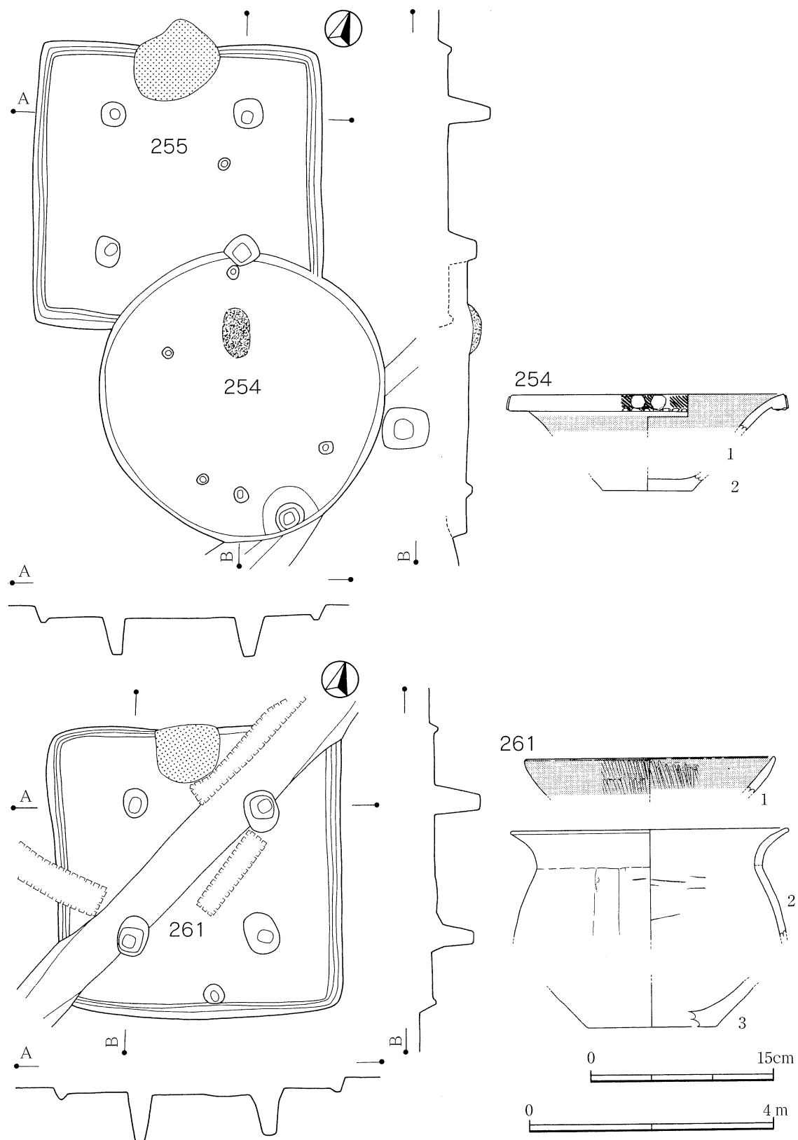
第104図 254・255・261号住居跡と254・261号住居跡出土土器
