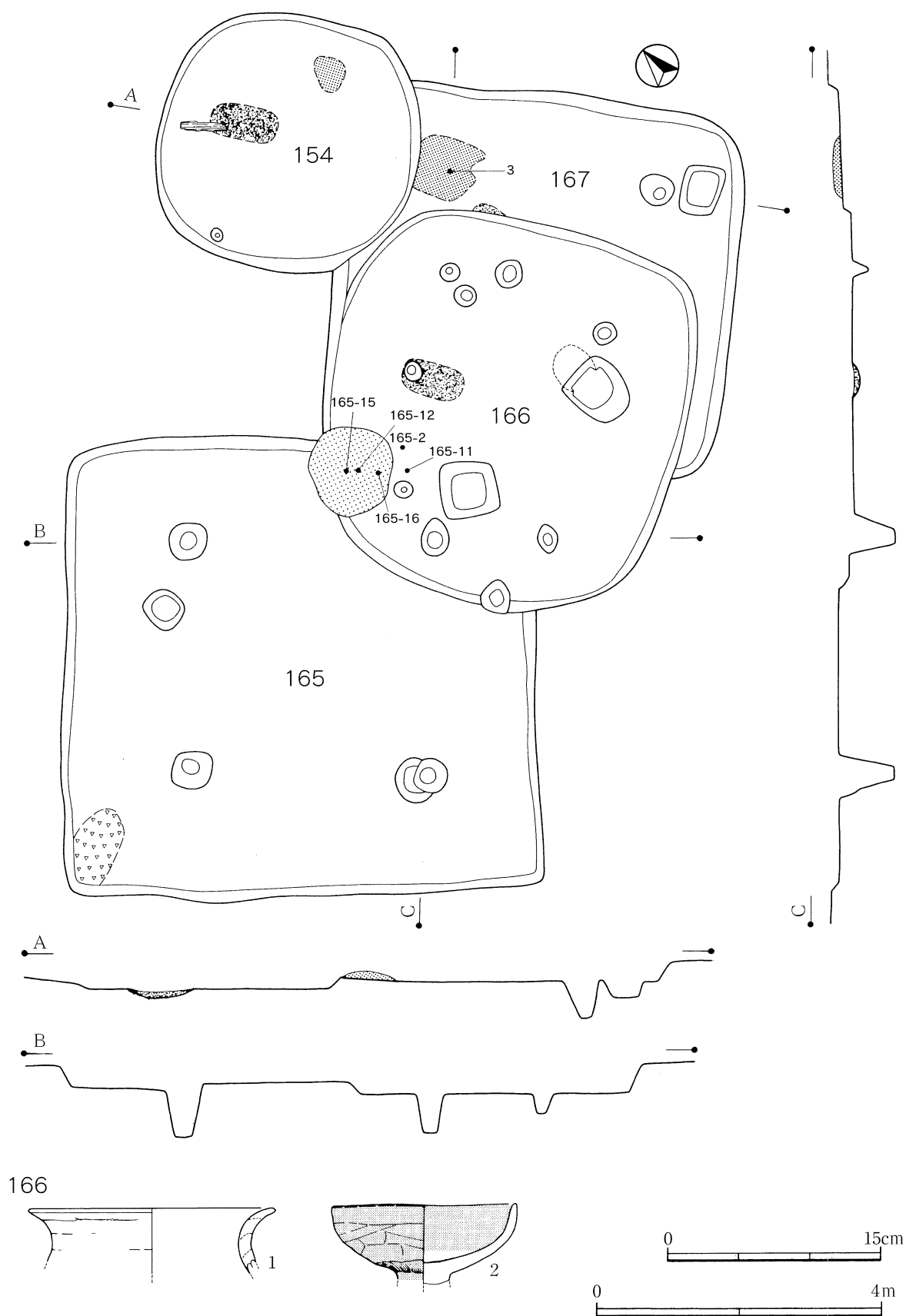
第80図 154・165～167号住居跡と166号住居跡出土土器
