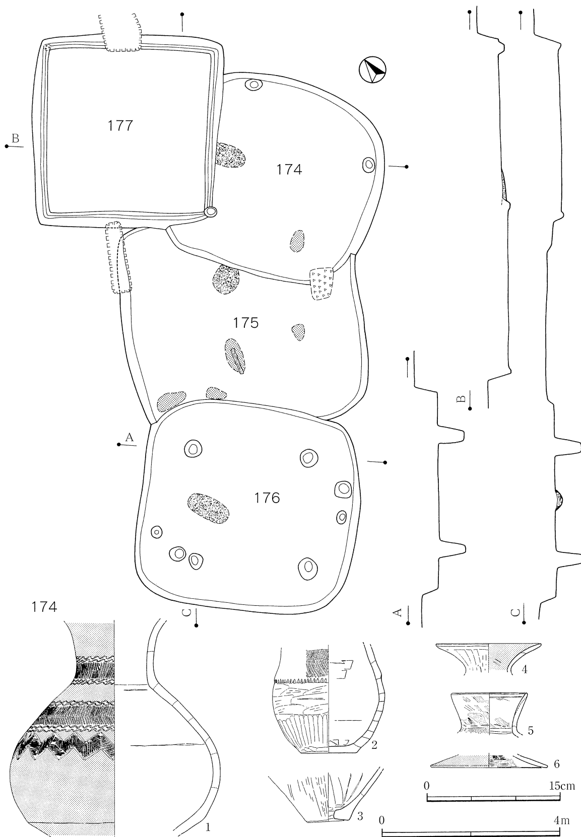
第86図 174～177号住居跡と174号住居跡出土土器
