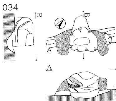
第130図 026・030・033・034・035・038・045号住居跡カマド
