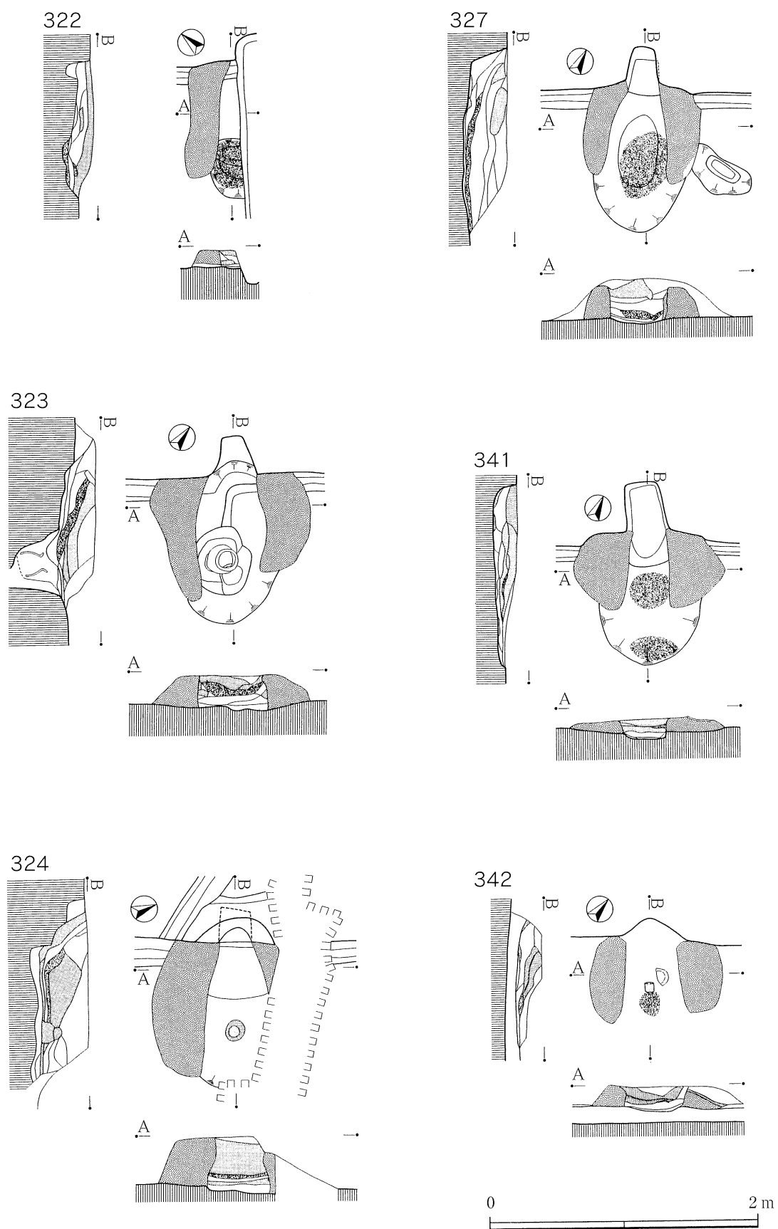
第141図 322・323・324・327・341・342号住居跡カマド
