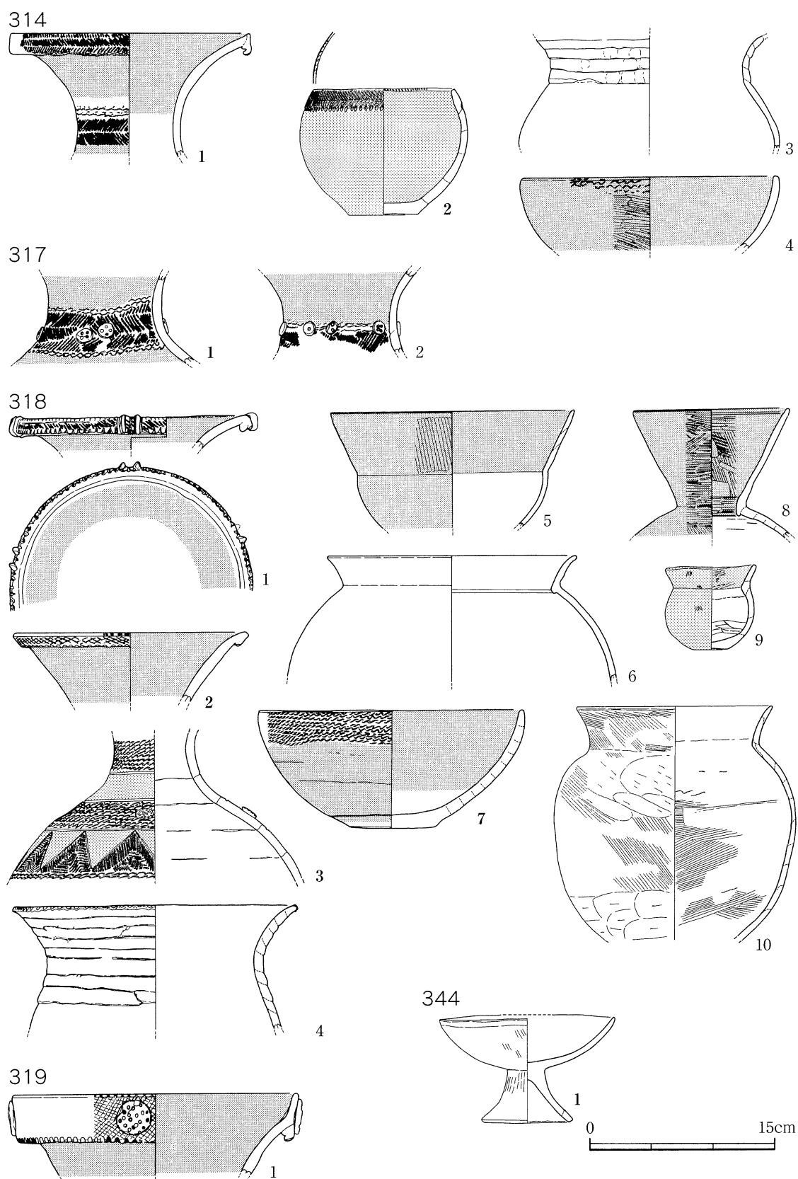
第119図 314・317~319・344号住居跡出土土器
