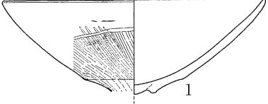
15号方形周溝墓
