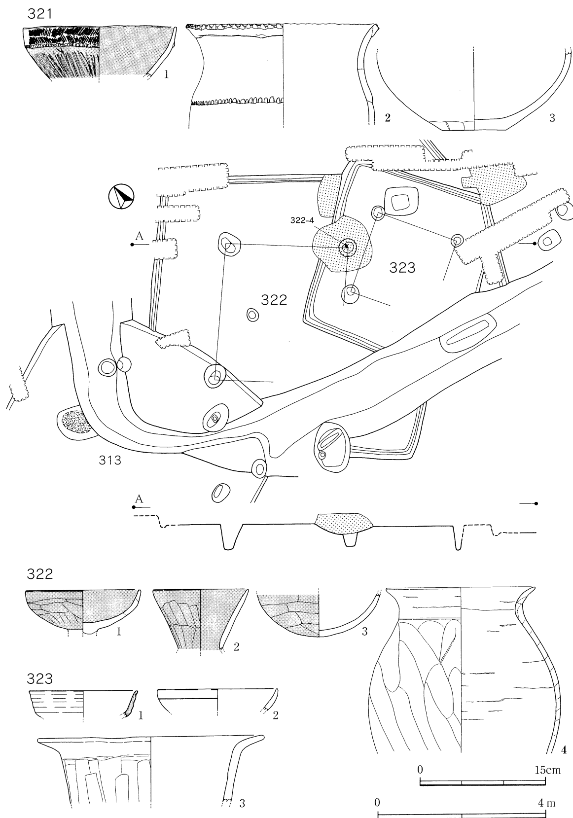
第121図 322・323号住居跡と321～323号住居跡出土土器
