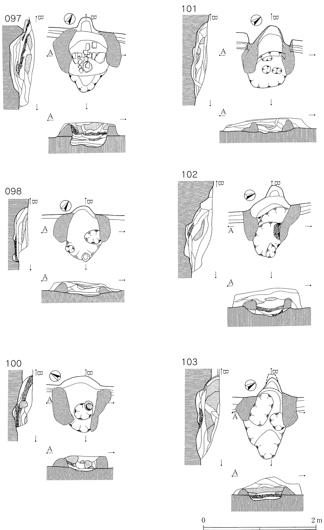
第133図 097・098・100・101・102・103号住居跡カマド
