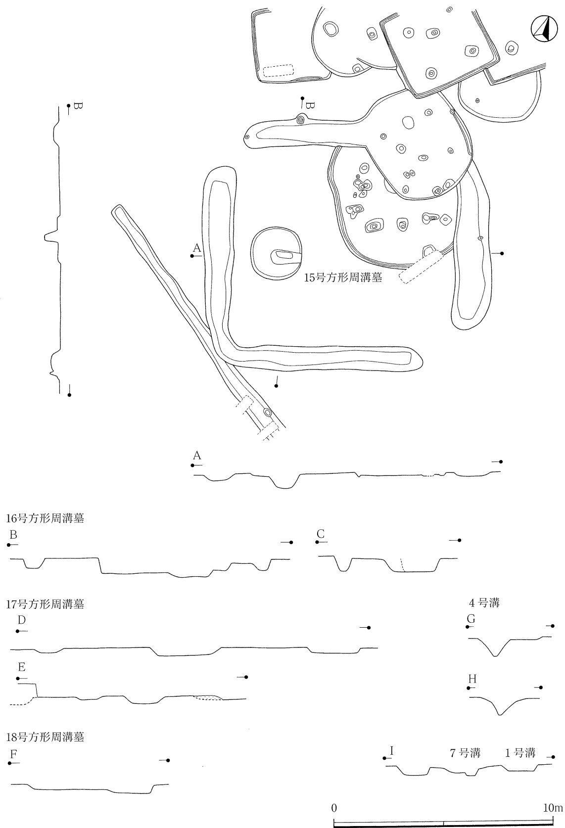
第162图 15号方形周溝墓
