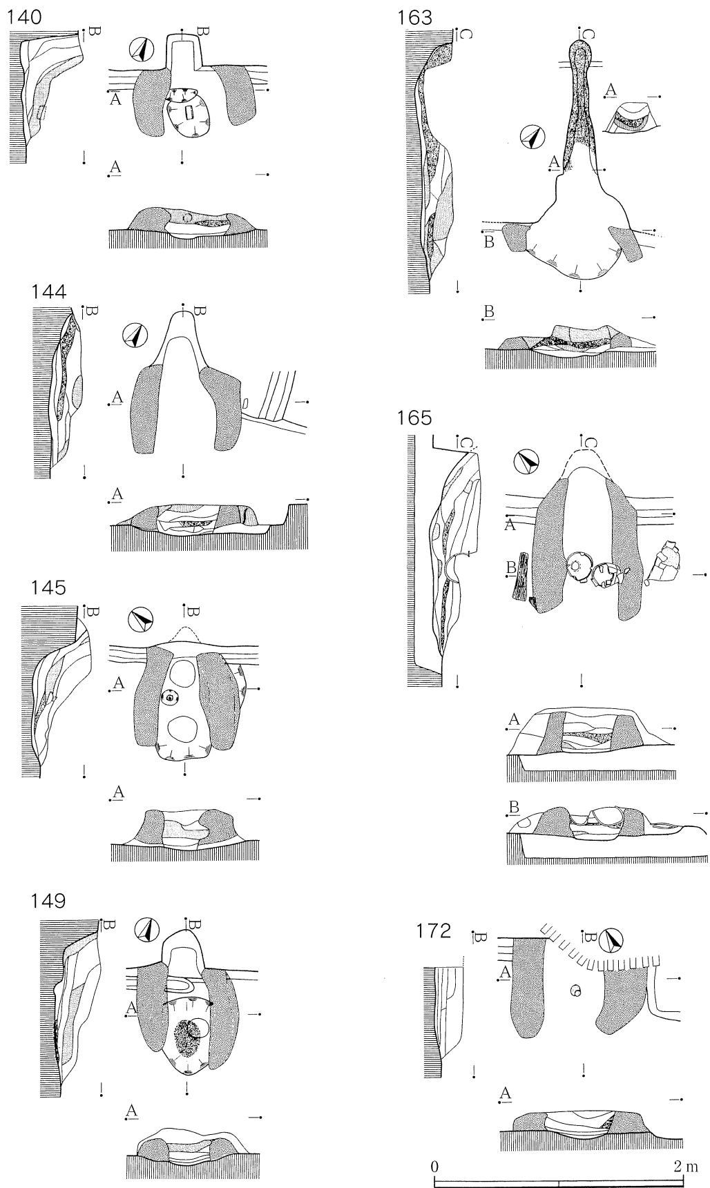
第136図 140・144・145・149・163・165・172号住居跡カマド
