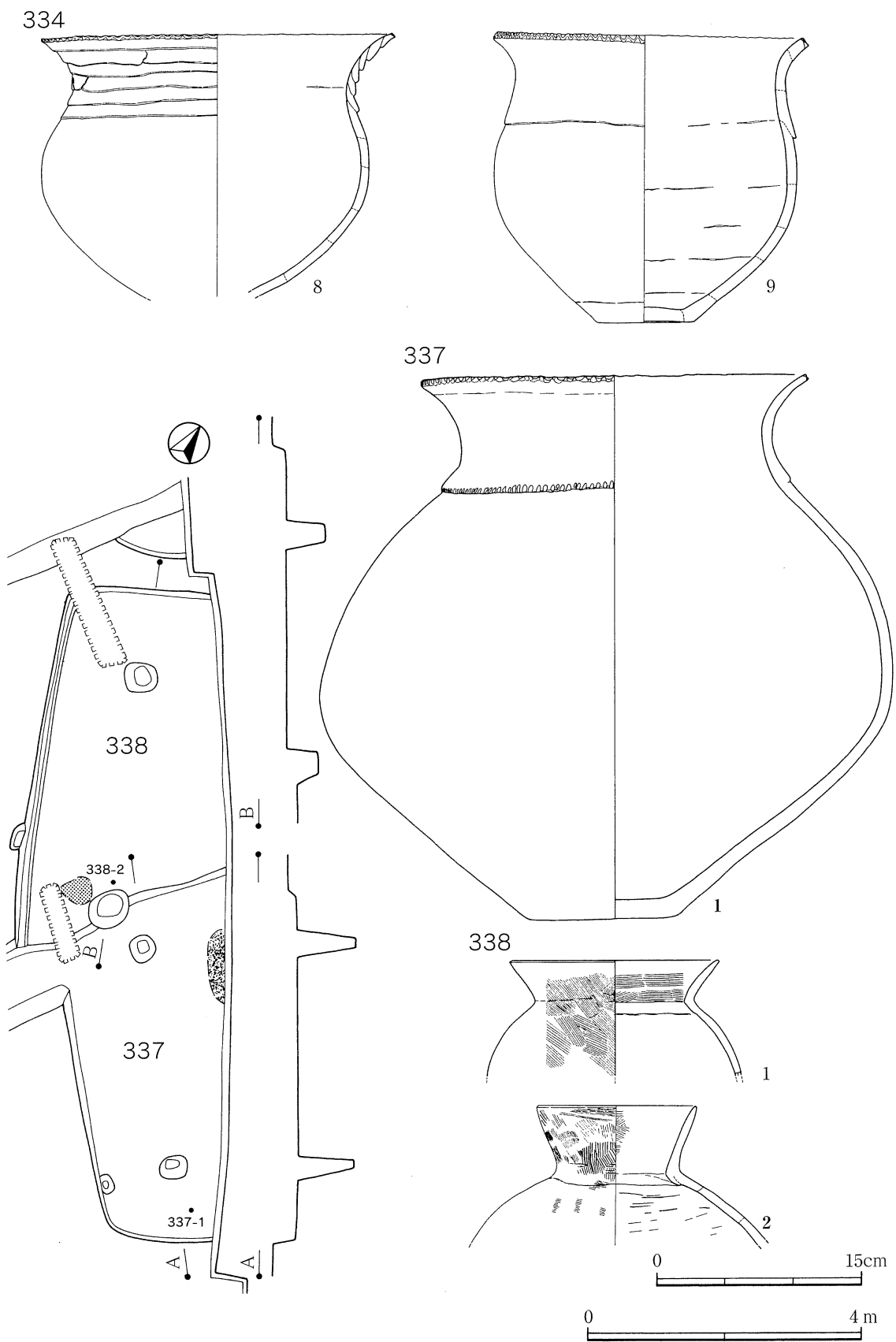
第126図 337・338号住居跡と334・337・338号住居跡出土土器
