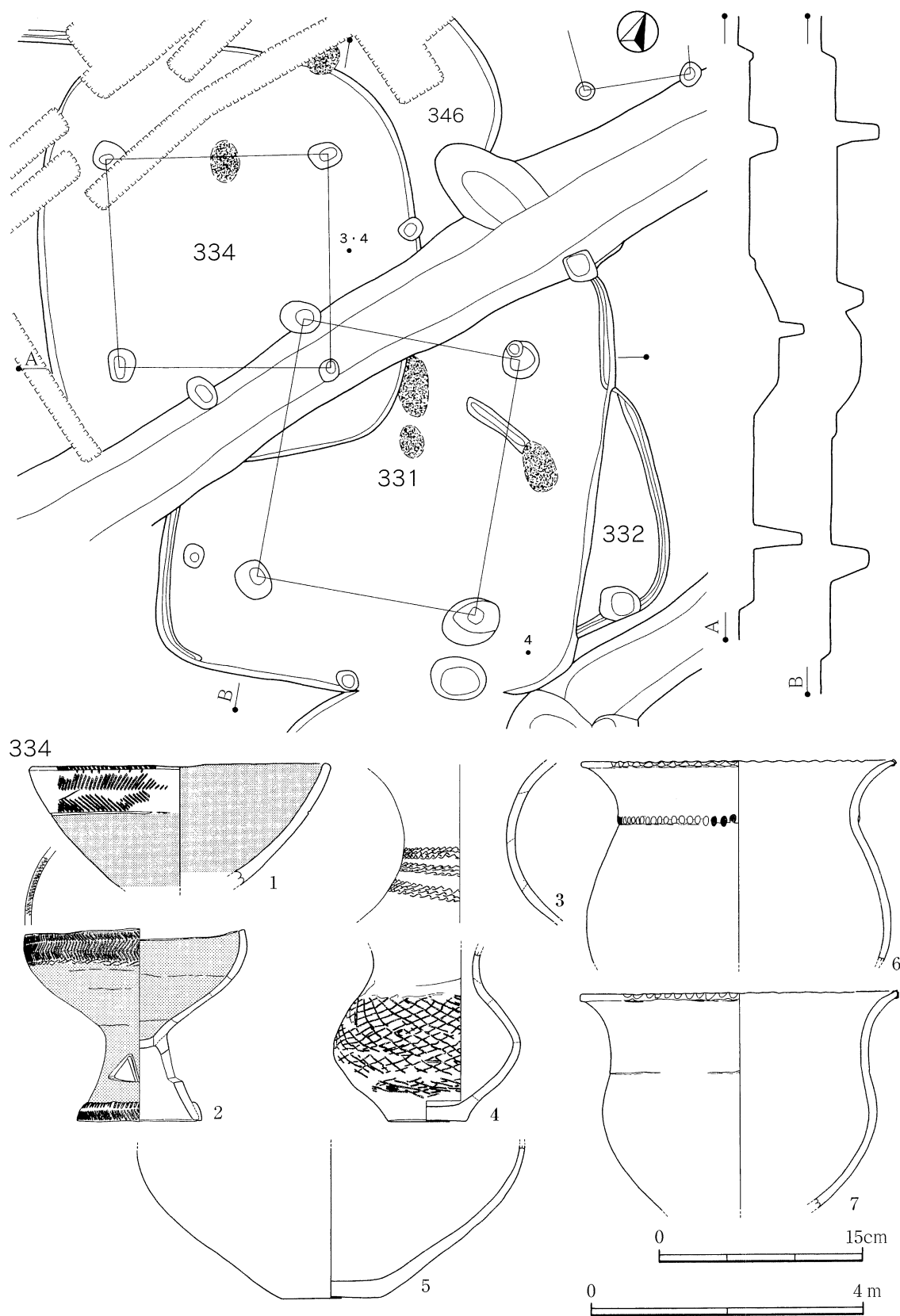
第125図 331・332・334号住居跡と334号住居跡出土土器
