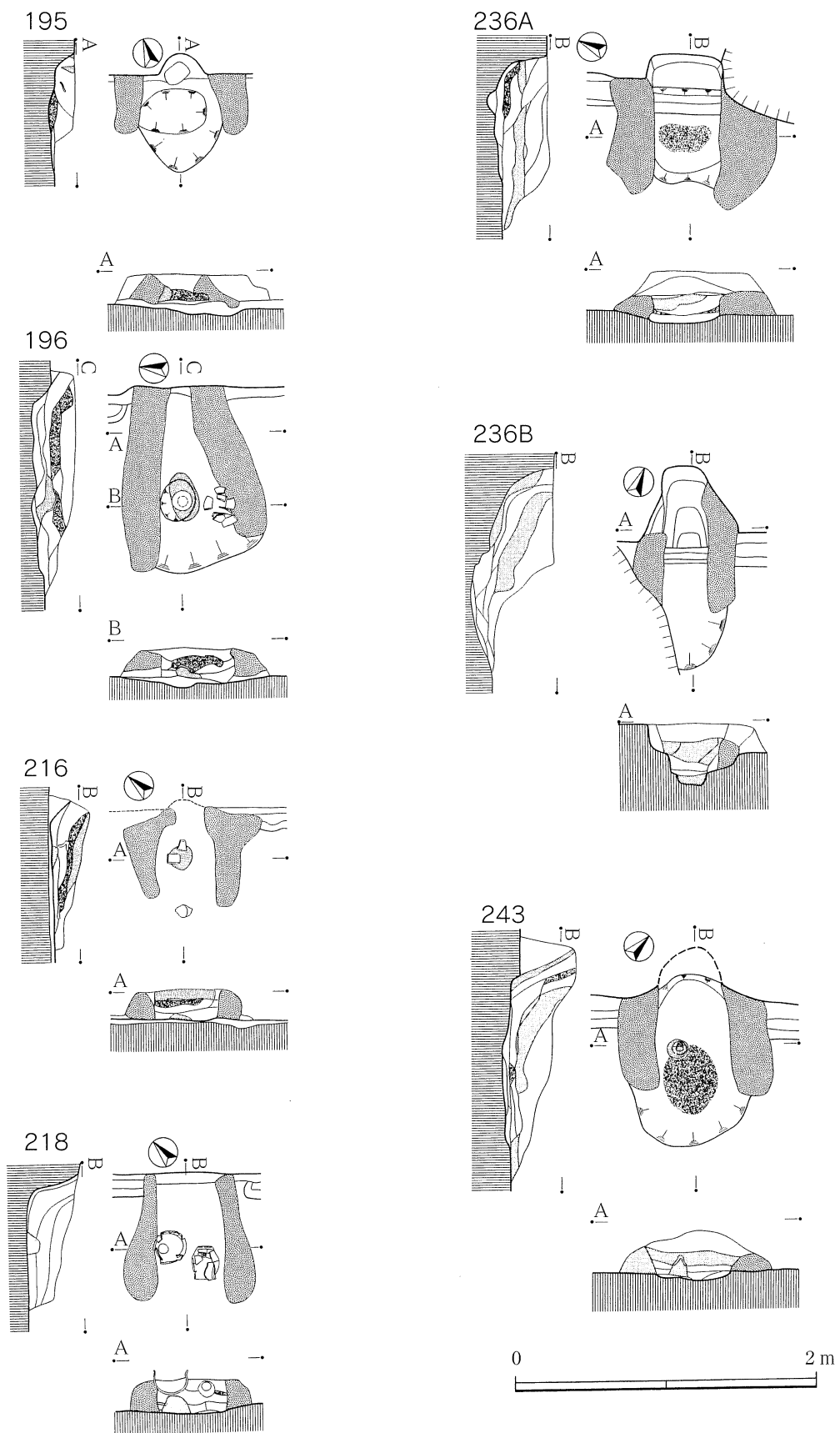
第138図 195・196・216・218・236A・236B・243号住居跡カマド
