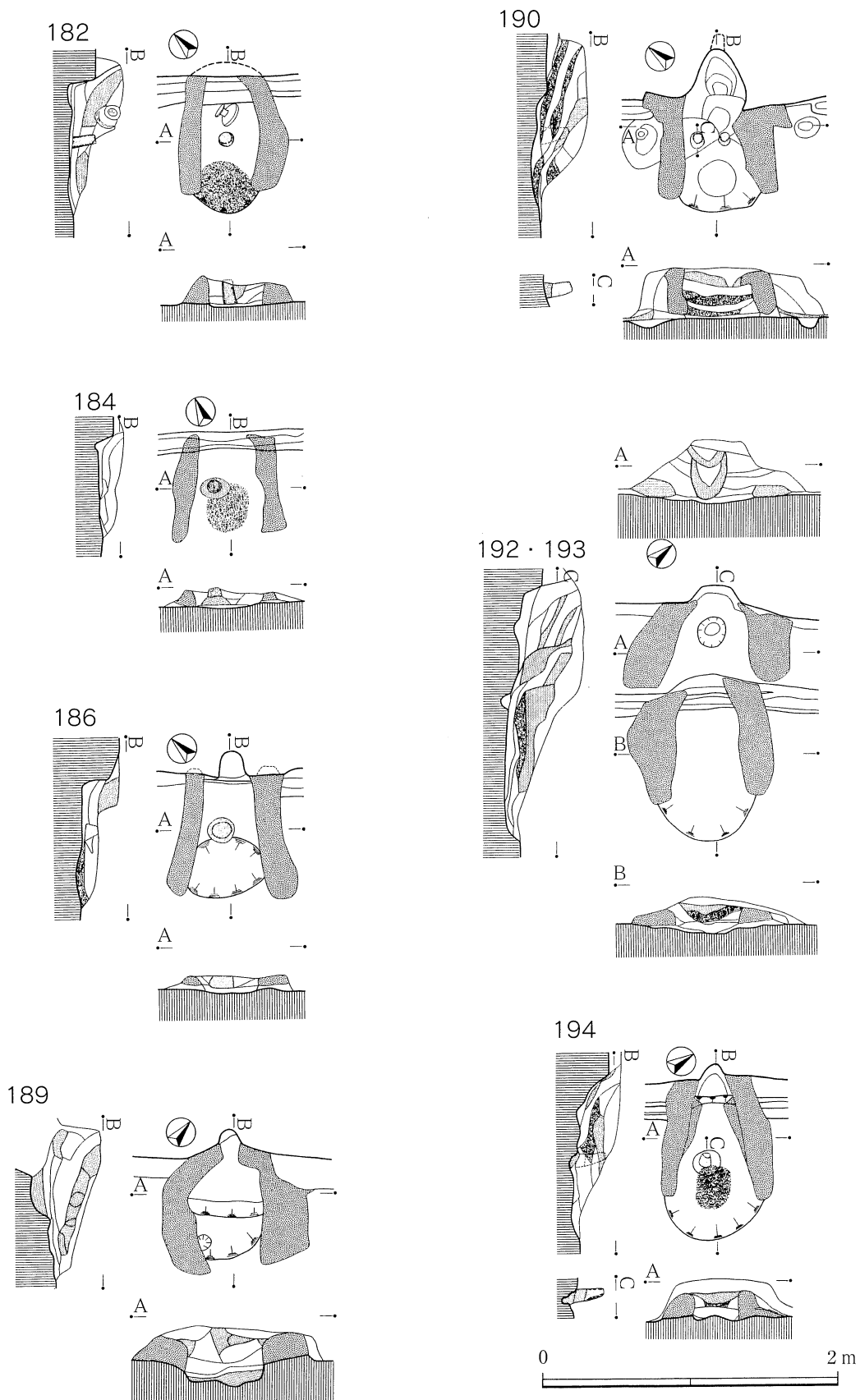
第137図 182・184・186・189・190・192・193・194号住居跡カマド
