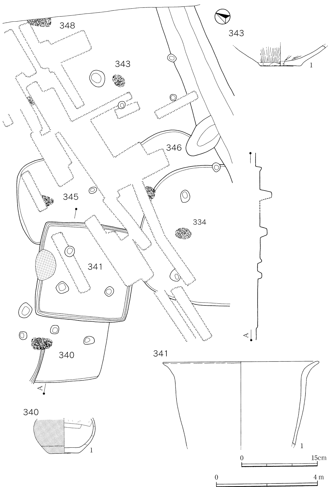
第127図 340・341・343・345・346・348号住居跡と340・341・343号住居跡出土土器
