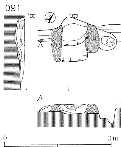
第132図 072B・073・076・079・081・085・091号住居跡カマド
