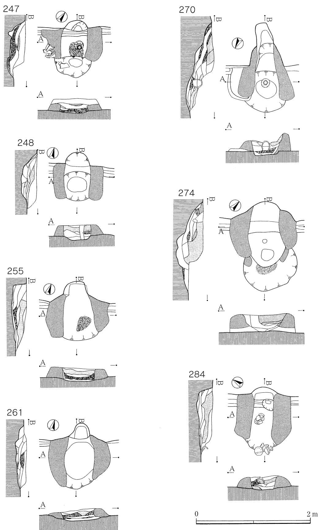
第139図 247・248・255・261・270・274・284号住居跡カマド
