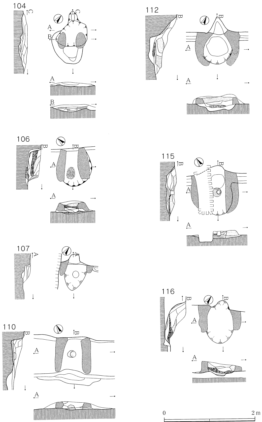
第134図 104・106・107・110・112・115・116号住居跡カマド
